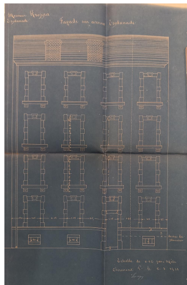
Élévation, 13 avenue d'Italie Repro. Félicie Fougère , Autr. auteur inconnu IVR84_20246300077NUCA
