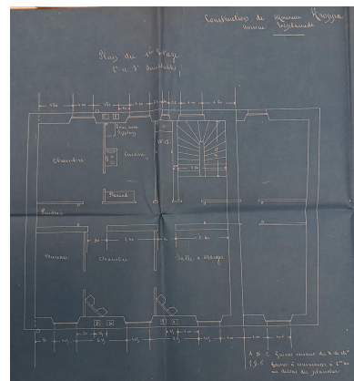
Plan des étages du n °13 avenue d'Italie Repro. Félicie Fougère , Autr. auteur inconnu IVR84_20246300078NUCA
