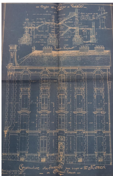
Coupe dans l'axe du vestibule et élévation principale, 1 rue d'Alsace Repro. Félicie Fougère , Autr. Louis Raynaud IVR84_20246300066NUCA
