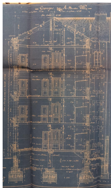
Coupe du 1 rue d'Alsace Repro. Félicie Fougère , Autr. Louis Raynaud IVR84_20246300065NUCA
