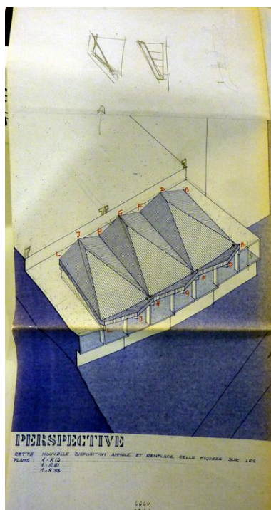
Etude pour la charpente de la salle à manger. Perspective / Atelier
