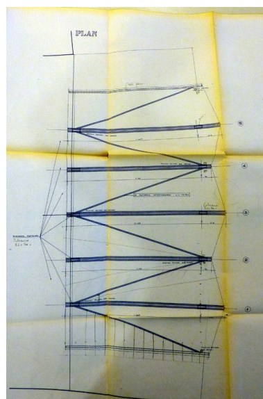
Etude pour la charpente de la salle à manger. Plan / Atelier d'Architecture en Montagne, mai 1974. (AD Savoie. 6J 1453) Phot. Jean-François Lyon-Caen IVR82_20127302319NUCA
