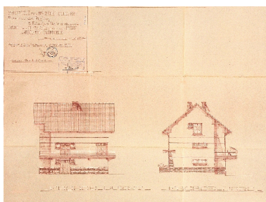
Elévations ouest et nord Repro. François Fouger IVR82_20097301323NUCB
