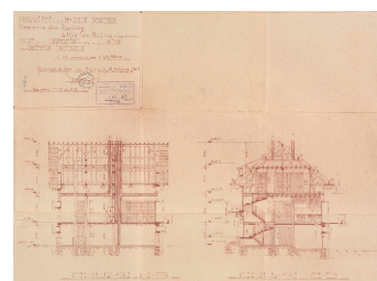
Coupes Repro. François Fouger IVR82_20097301237NUCB
