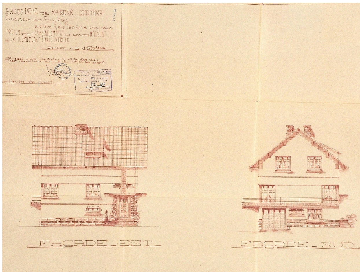
Elévations est et sud
