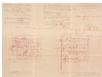
Plans de situation, du sous-sol et du 1er étage Repro. François Fouger IVR82_20097301236NUCB
