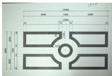
Maquette : plan coté par E. Louisgrand, 2005 (A Région Auvergne-Rhône-Alpes site de Clermont-Ferrand, 747 WR 30) Repro. Catherine Guégan, Autr. Emmanuel Louisgrand IVR84_20254300014NUC
