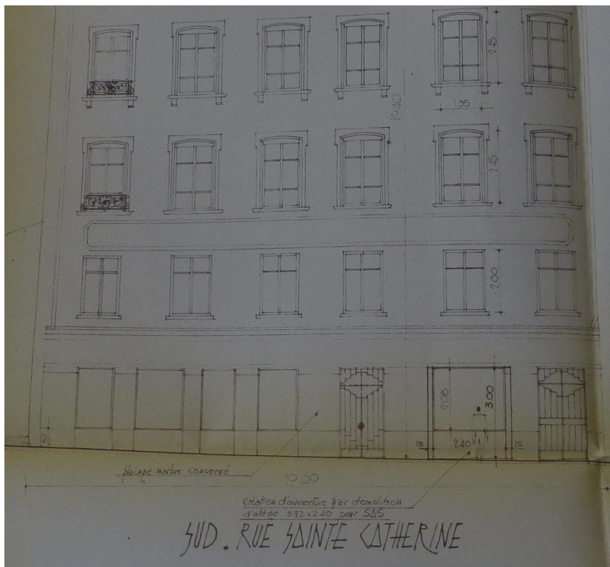
Façade sud détail rez-de-chaussée de l'Imprimerie Nouvelle Lyonnaise, 1981 (ACL : 405W008)
