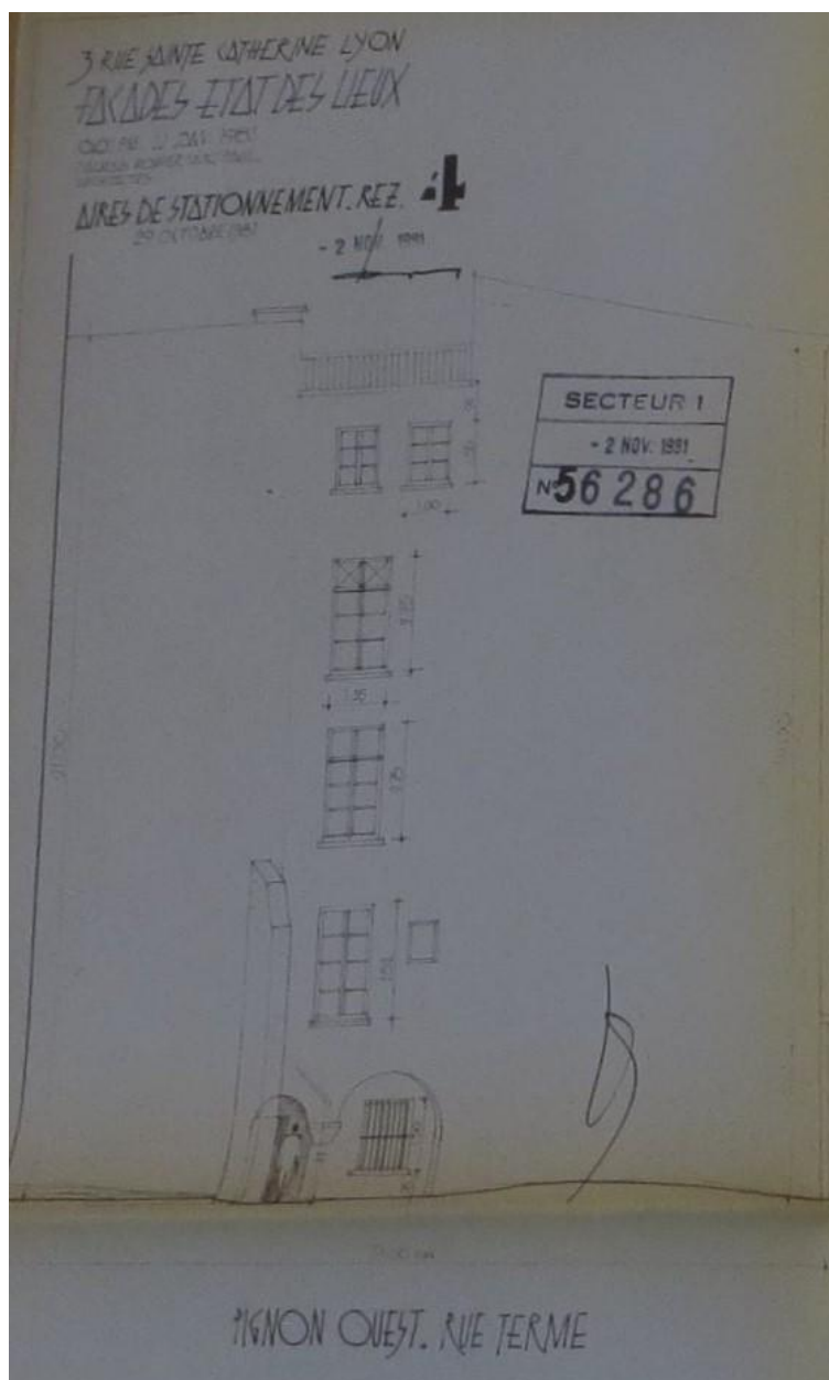
Façade pignon ouest rue Terme de l'Imprimerie Nouvelle Lyonnaise, 1981 (ACL : 405W008)
