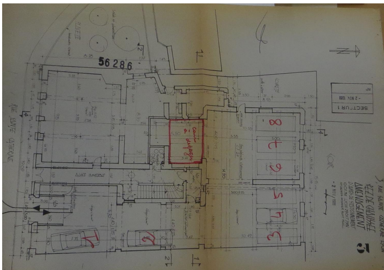
Projet parking, plan du rez-de-chaussée, 1981 (ACL : 405W008)
