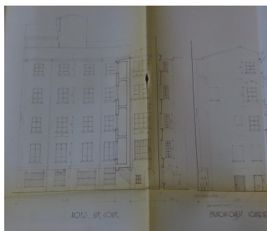
Façade nord de l'Imprimerie Nouvelle Lyonnaise, 1981 (ACL : 405W008) Phot. Nadine Halitim-Dubois IVR84_20246900679NUCA
