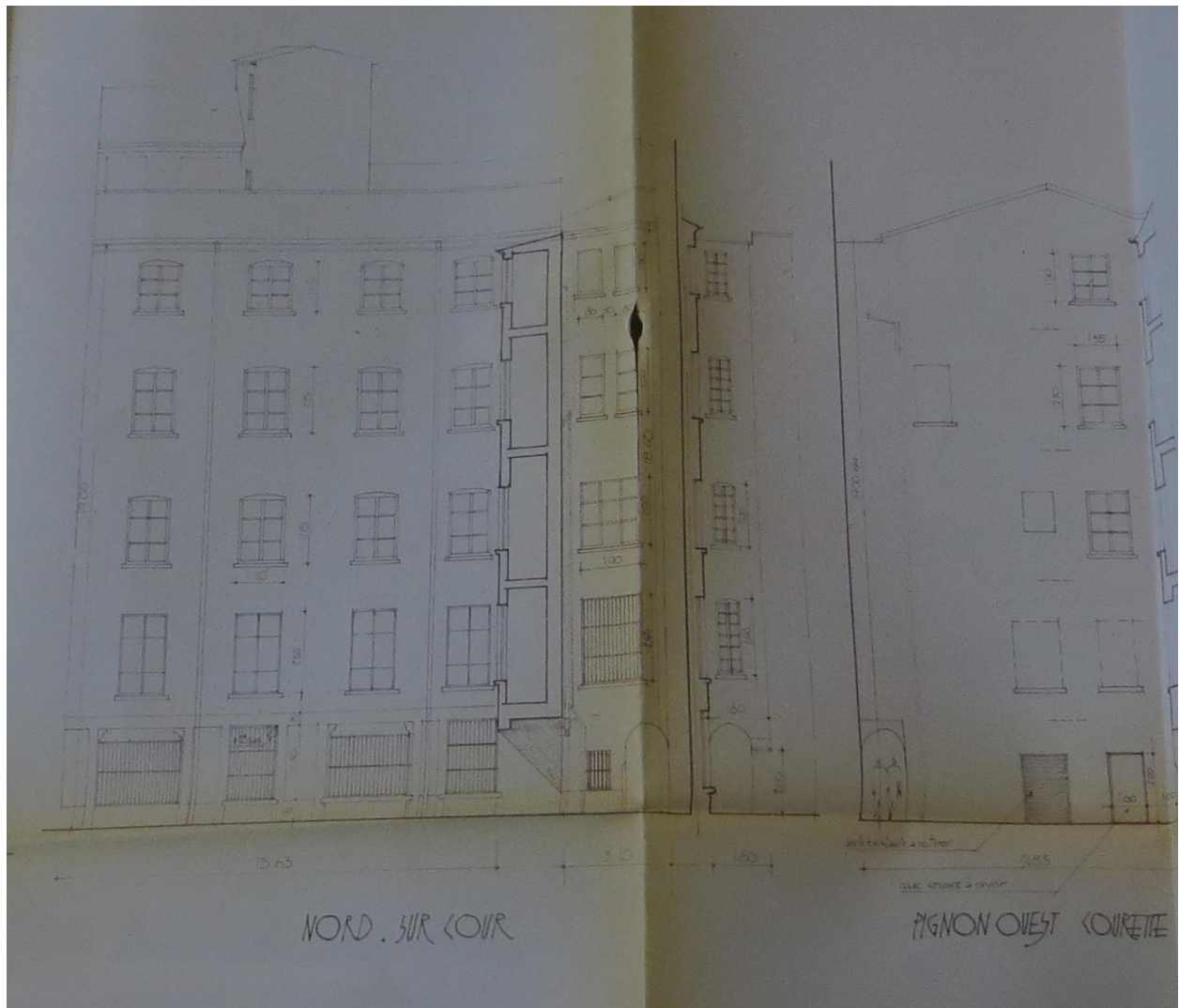
Façade nord de l'Imprimerie Nouvelle Lyonnaise, 1981 (ACL : 405W008)
