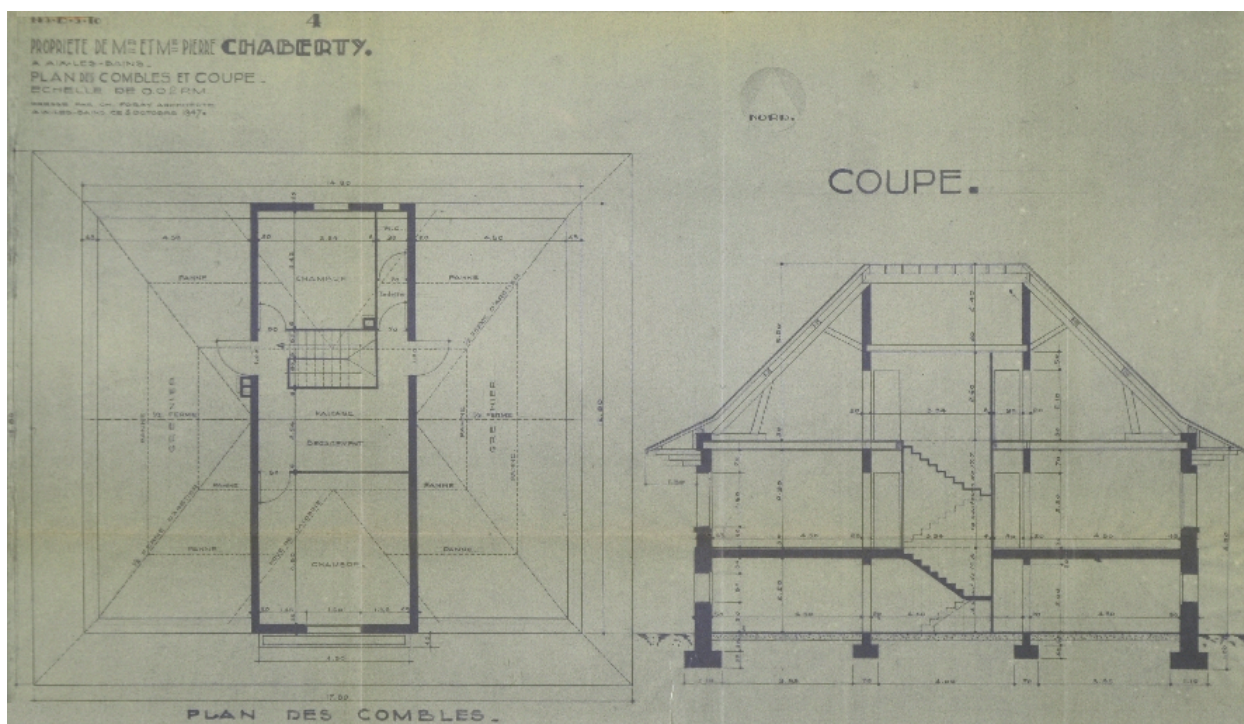
Plan des combles et coupe
