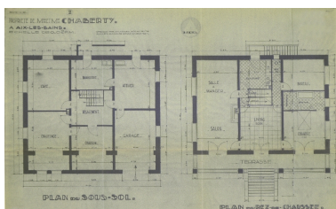
Plans du sous-sol et du rez-de-chaussée Repro. François Fouger IVR82_20127300382NUCB
