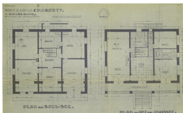
Plans du sous-sol et du rez-de-chaussée Repro. François Fouger IVR82_20127300382NUCB
