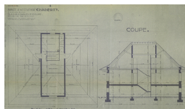
Plan des combles et coupe Repro. François Fouger IVR82_20127300384NUCB
