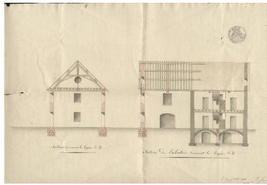
Coupes Repro. François Fouger IVR82_20077300836NUCB
