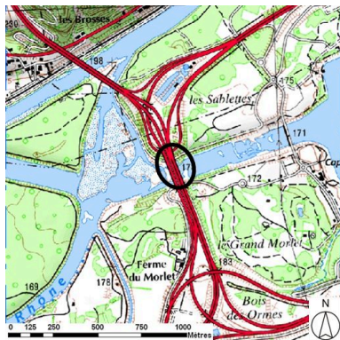
Plan de situation (sur fond de SCAN25(R) (C) IGN-2008 (C) Région Rhône-Alpes Licence n°2008-CISE27-1010) Dess. S. Delétoille IVR82_20106907526NUD
