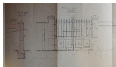
Construction de murs de clôture avec grilles et aménagement des allées intérieures, plan et profils, 1924 (AC Savigneux. M 3). Autr. Rolin, Repro. Elisabeth Dandel IVR84_20190100360NUCAB
