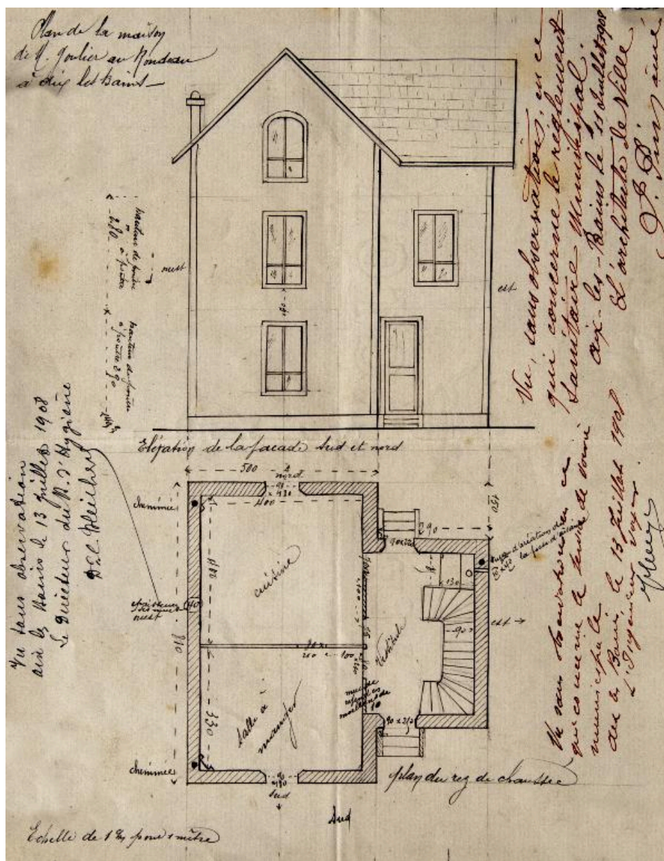
Plan du rdc et façade principale, 1908
