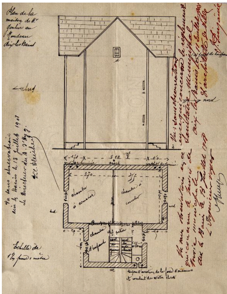
Plan du 1er étage et façade postérieure, 1908
