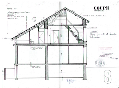
Coupe après transformation Repro. François Fouger IVR82_20077300863NUCB
