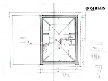
Plan du comble après transformation Repro. François Fouger IVR82_20077300862NUCB
