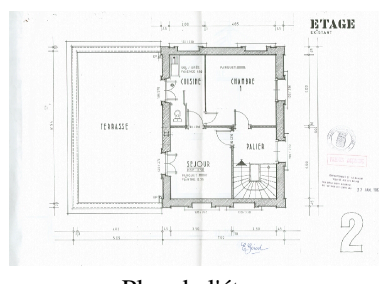
Plan de l'étage Repro. François Fouger IVR82_20077300857NUCB
