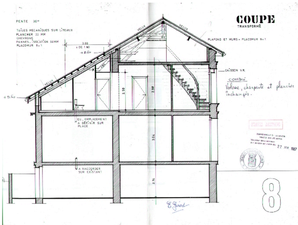
Coupe après transformation
