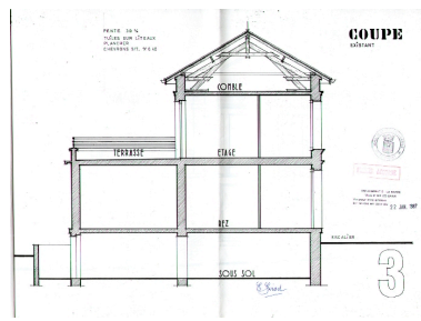
Coupe Repro. François Fouger IVR82_20077300858NUCB
