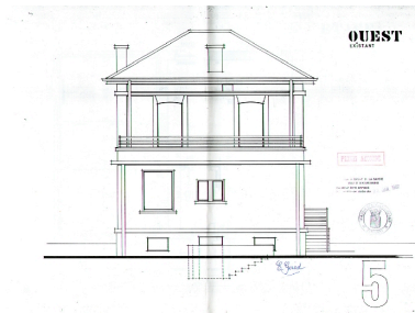
Elévation occidentale Repro. François Fouger IVR82_20077300860NUCB
