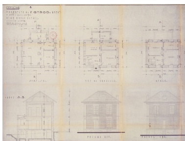
Plans, coupe et élévations Repro. François Fouger IVR82_20077300660NUCB
