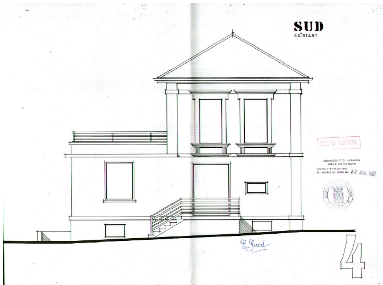
Elévation sud
