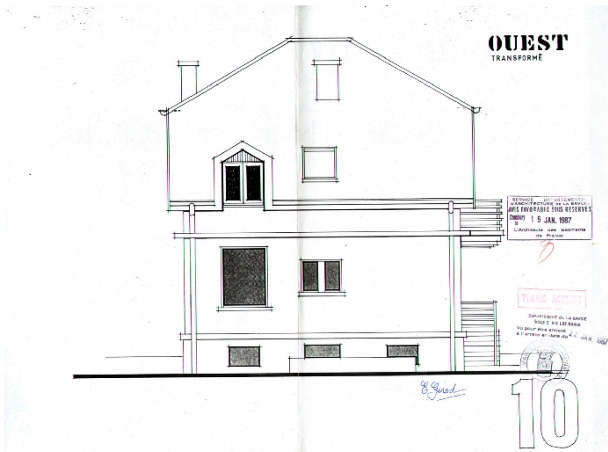
Elévation occidentale après transformation
