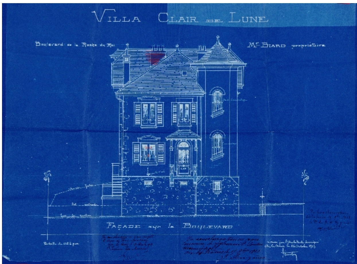
Elévation principale
