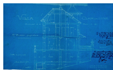
Coupe Repro. François Fouger IVR82_20117300226NUCB
