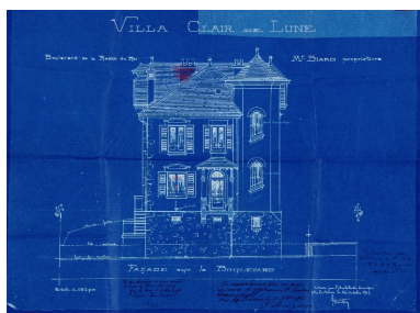
Elévation principale Repro. François Fouger IVR82_20117300228NUCB
