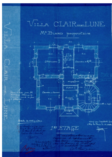
Plan du 1er étage Repro. François Fouger IVR82_20117300227NUCB
