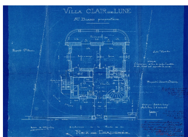
Plan du rez-de-chaussée Repro. François Fouger IVR82_20117300229NUCB
