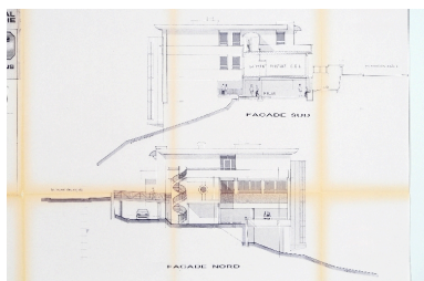
Elévations sud et nord Repro. François Fouger IVR82_20107300911NUCB
