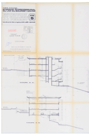
Coupes AA et BB Repro. François Fouger IVR82_20107300909NUCB
