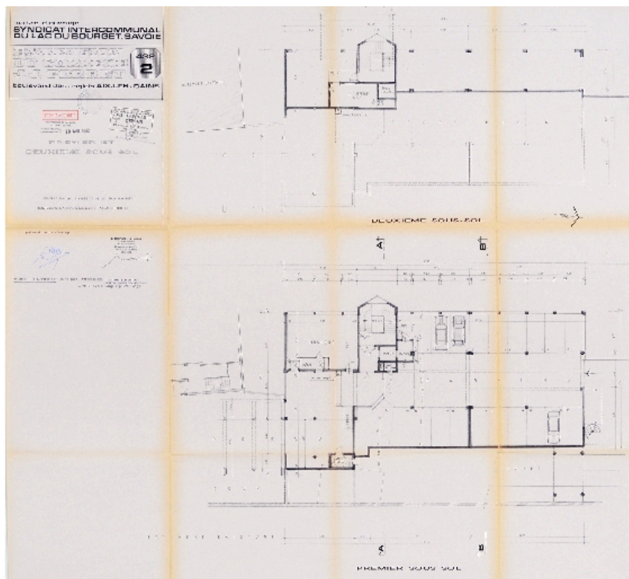
Plans des 1er et 2e sous-sol
