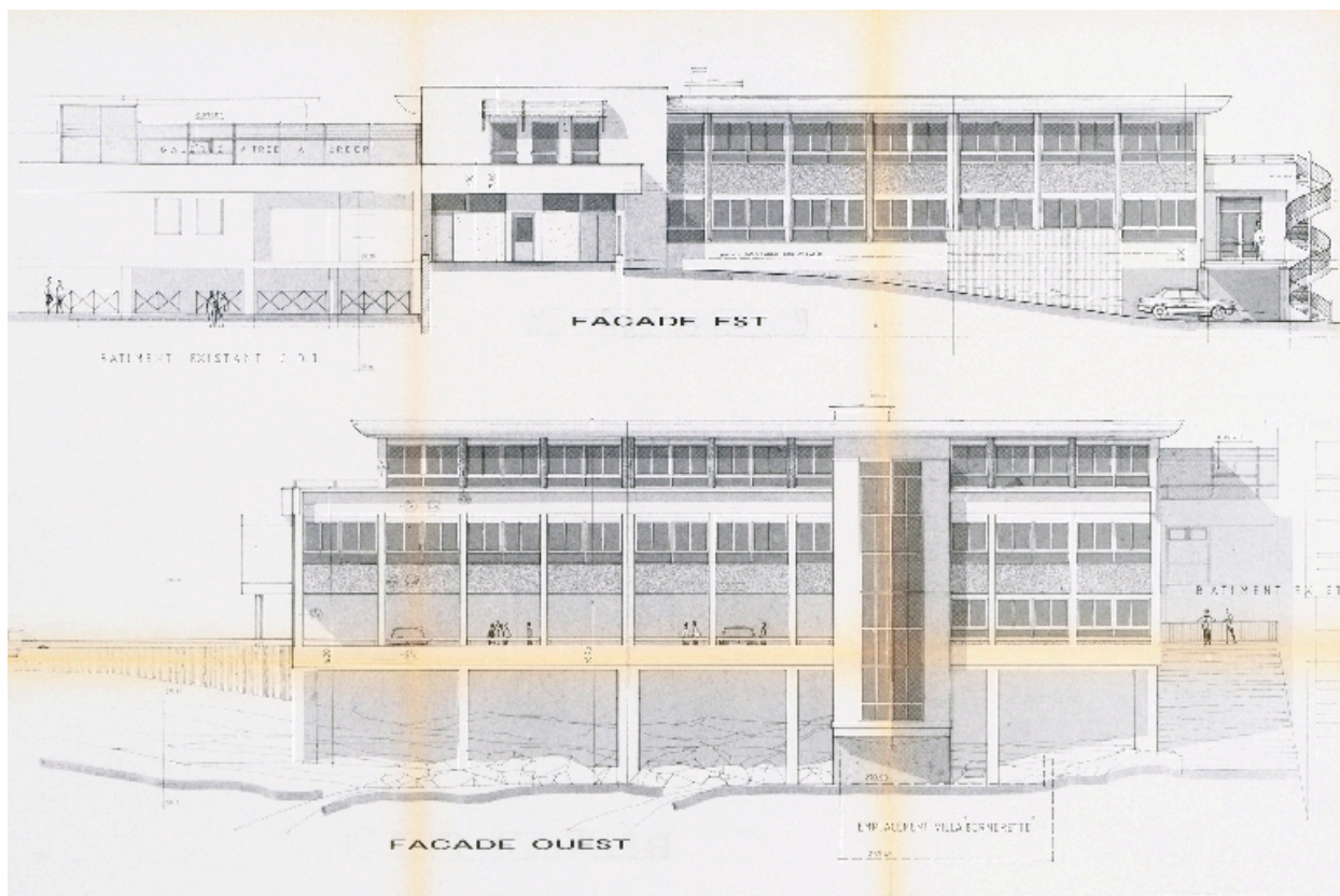
Elévations est et ouest
