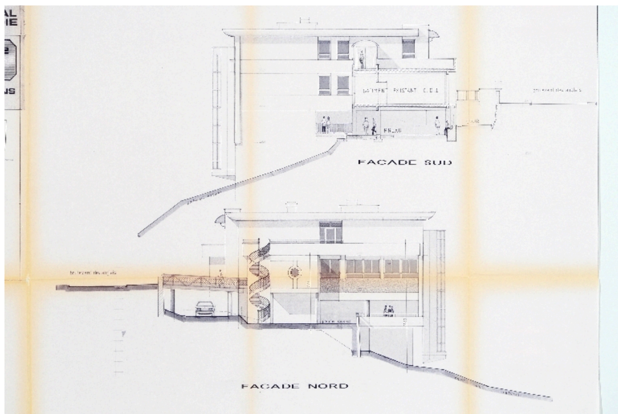
Elévations sud et nord
