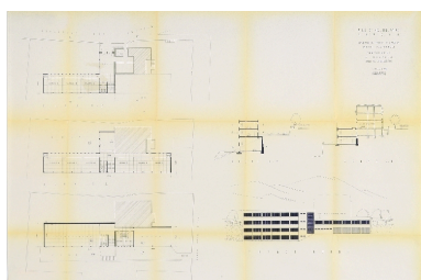
Plans, coupes et élévations Repro. François Fouger IVR82_20107300904NUCB
