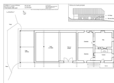
Plan du rez-de-chaussée surélevé. Dess. André Céréza IVR84_20177401005NUD
