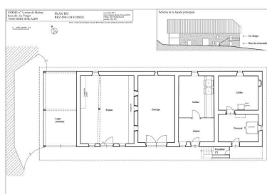
Plan de l'étage de soubassement. Dess. André Céréza IVR84_20177401004NUD
