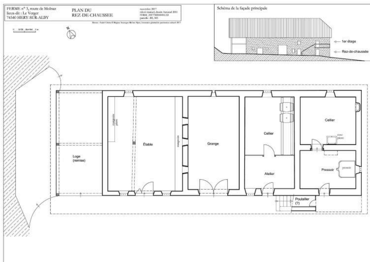
Plan de l'étage de soubassement.
