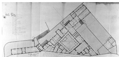
N° 3. Plan des bâtiments de l'hospice de l'Antiquaille (...), faisant rez- de-chaussée du côté de l'entrée principale, premier étage du côté nord, et une partie côté orient faisant deuxième étage, par Perenciol, 1811 Phot. Jean-Marie Refflé IVR82_20016901318P
