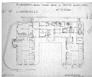
Achèvement du nouveau bâtiment [18] destiné au service des malades. [1] Rez de chaussée, 1903 Phot. Jean-Marie Refflé IVR82_20016901305P
