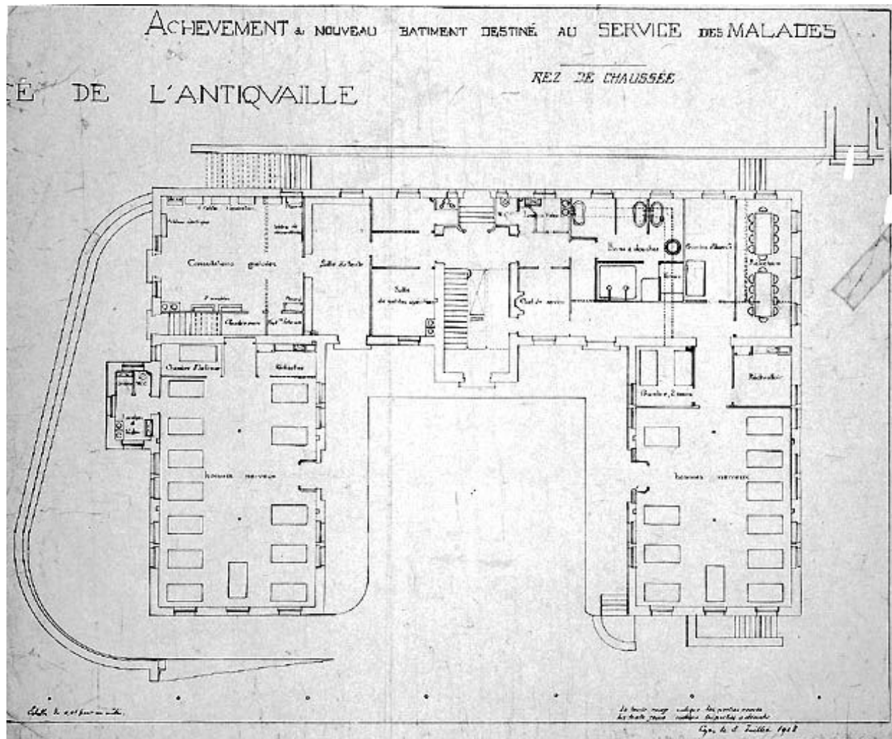
Achèvement du nouveau bâtiment [18] destiné au service des malades. [1] Rez de chaussée, 1903
