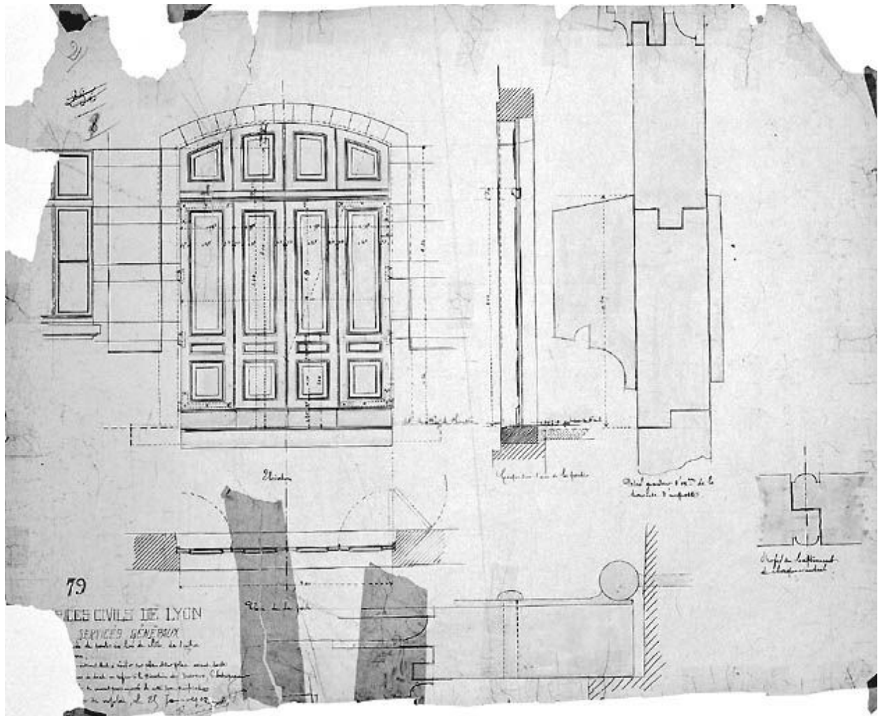
Bâtiment 18, vantaux en chêne des portes des ailes, plans, coupe, élévation, 1902
