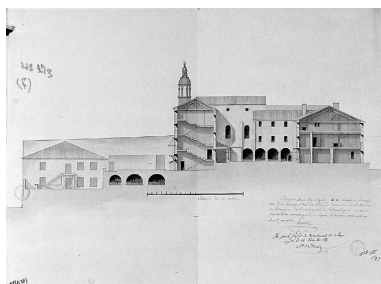
Coupe sur la ligne A.B. tracée, en rouge, sur le troisième plan du rez- de-chaussée du bâtiment de l'hospice de l'Antiquaille, par Perenciol, 1811 Phot. Jean-Marie Refflé
