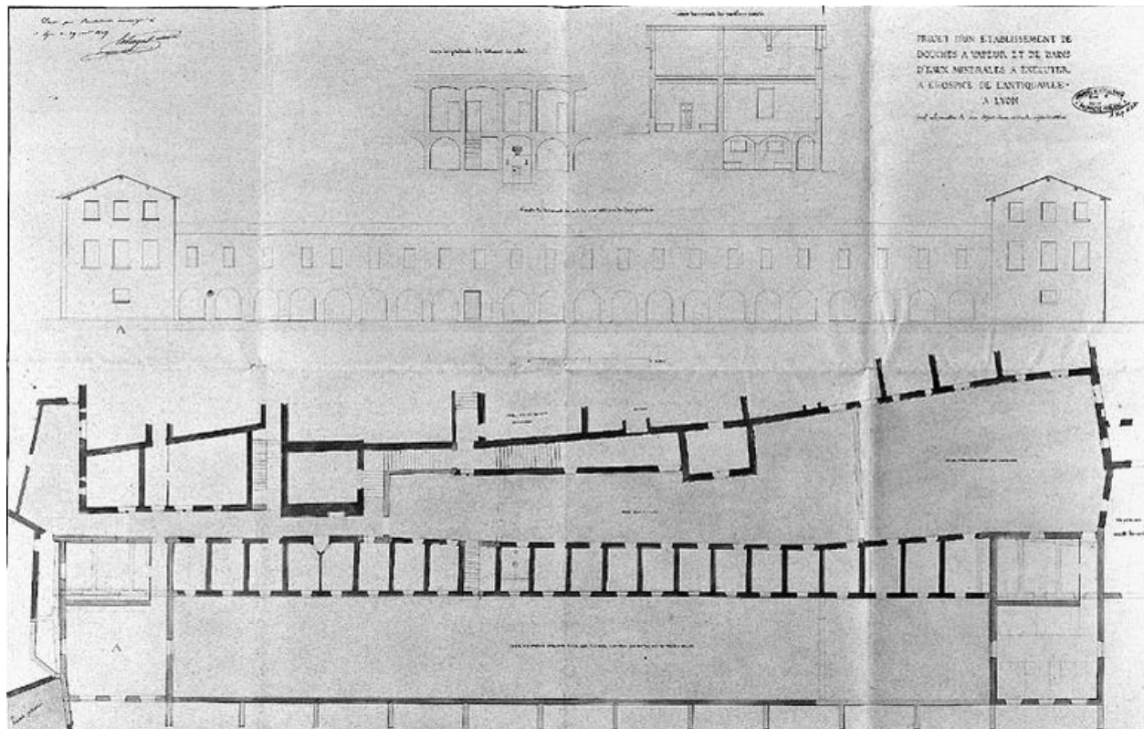
Projet d'un établissement de douches à vapeur et de bains d'eaux minérales à exécuter à l'hospice de l'Antiquaille à Lyon [au bout du bâtiment des Loges], par Exbrayat, 1839
