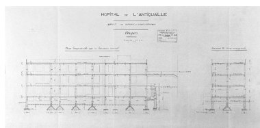
Hôpital de l'Antiquaille. Service de dermato-syphiligraphy [bâtiment 17]. 4. Coupes, 1936 Phot. Jean-Marie Refflé IVR82_20026900656P
