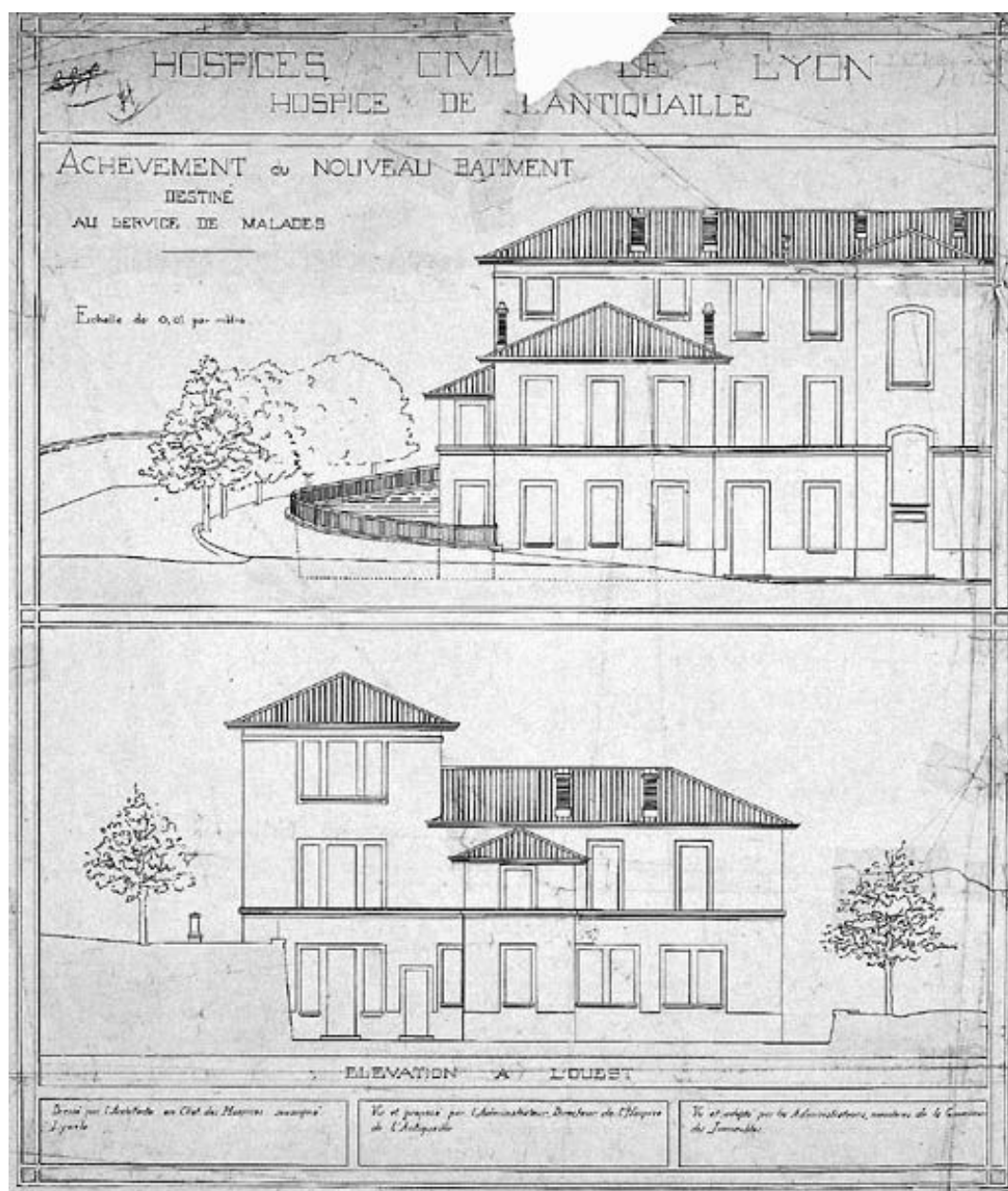
Achèvement du nouveau bâtiment [18] destiné au service des malades. [Elévation sud, moitié gauche]. Elévation à l'ouest, 1903
