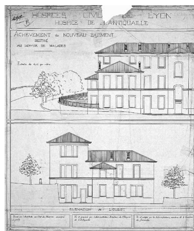
Achèvement du nouveau bâtiment [18] destiné au service des malades. [Elévation sud, moitié gauche]. Elévation à l'ouest, 1903 Phot. Jean-Marie Refflé IVR82_20016901306P
