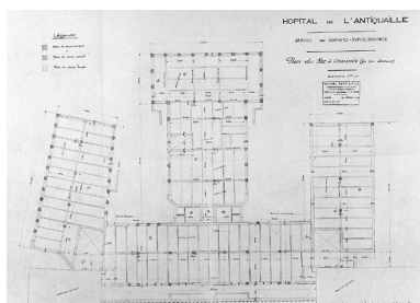
Hôpital de l'Antiquaille. Service de dermato-syphiligraphy [bâtiment 17]. 2. Plan du rez-de-chaussée (vue par dessous), 1936 Phot. Jean-Marie Refflé IVR82_20026900655P
