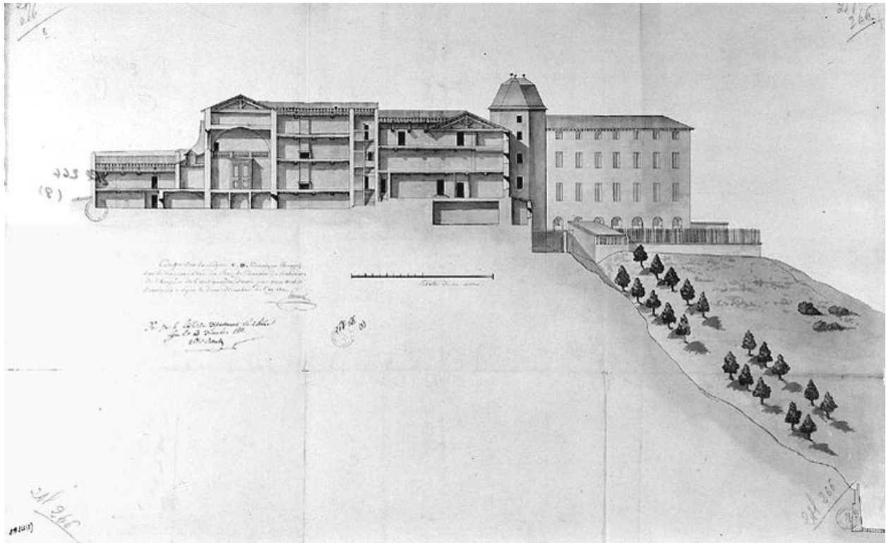
Coupe sur la ligne C.D. tracée, en rouge, sur le troisième plan du rez-de-chaussée du bâtiment de l'hospice de l'Antiquaille, par Perenciol, 1811
