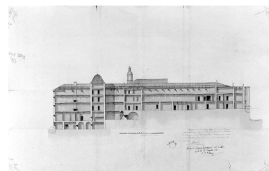
Coupe sur la ligne E.F. tracée, en rouge, sur le troisième plan du rez- de-chaussée du bâtiment de l'hospice de l'Antiquaille, par Perenciol, 1811 Phot. Jean-Marie Refflé
