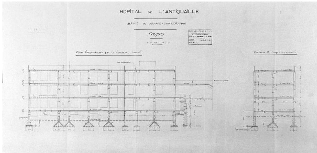
Hôpital de l'Antiquaille. Service de dermato-syphiligraphie [bâtiment 17]. 4. Coupes, 1936
