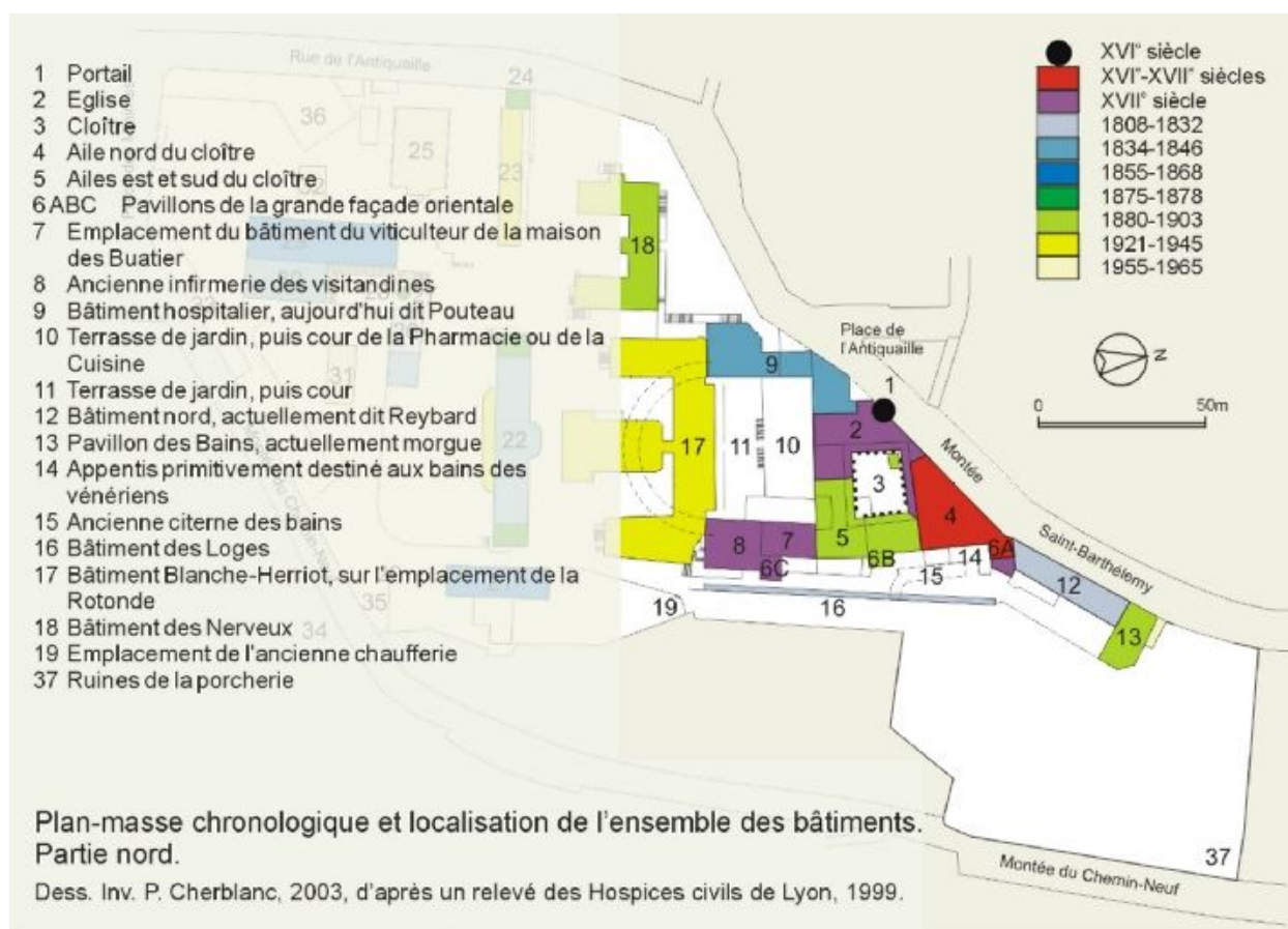
Plan-masse chronologique et localisation de l'ensemble des bâtiments, détail de la moitié nord avec légende
