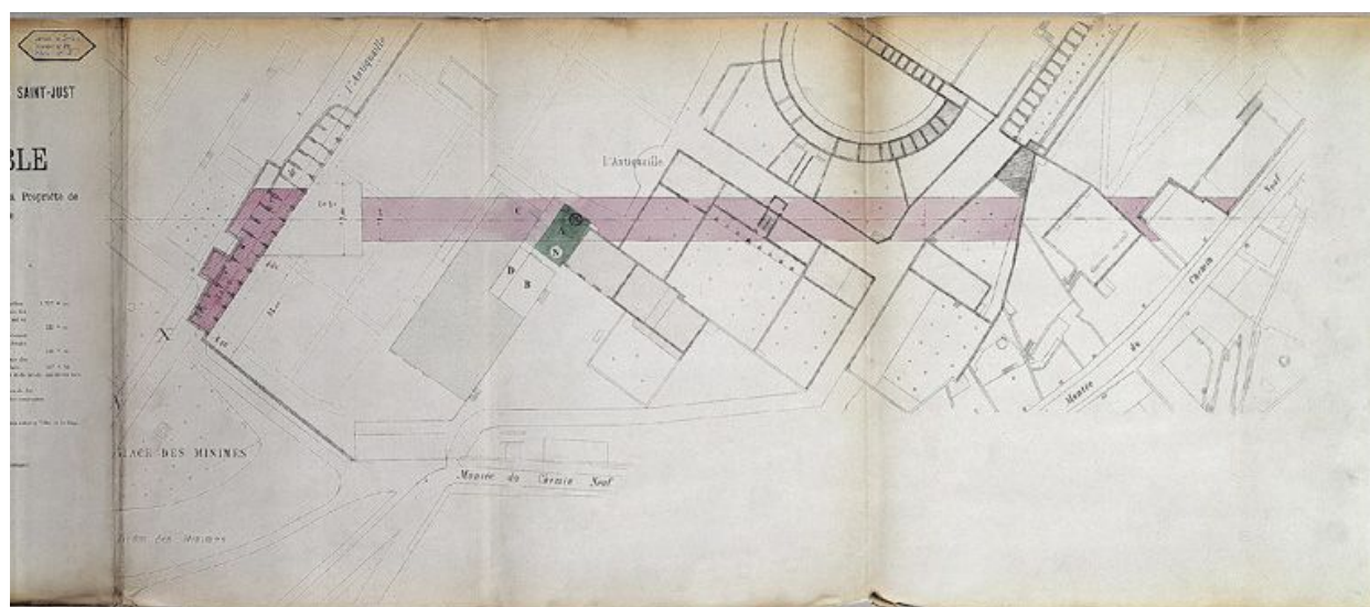
Chemin de fer de Lyon à Fourvière et à Saint-Just. Plan d'ensemble des terrains expropriés et dommages causés à la propriété de l'Antiquaille, appartenant à la ville, par Gobin, 1874
