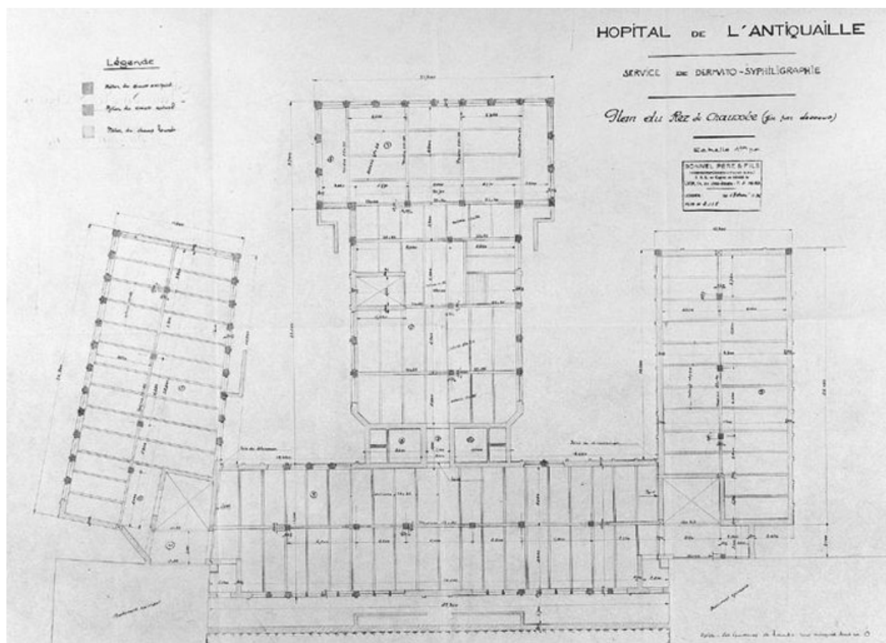
Hôpital de l'Antiquaille. Service de dermato-syphiligraphie [bâtiment 17]. 2. Plan du rez-de-chaussée (vue par dessous), 1936
