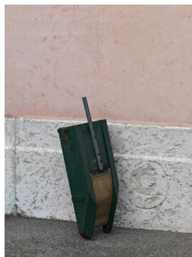
Drague à main et à manche utilisée pour les sédiments supérieurs Phot. Eric Dessert IVR82_20126901334NUCA
