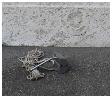
Benne type pince à sucre "Van Veen" Phot. Eric Dessert IVR82_20126901341NUCA
