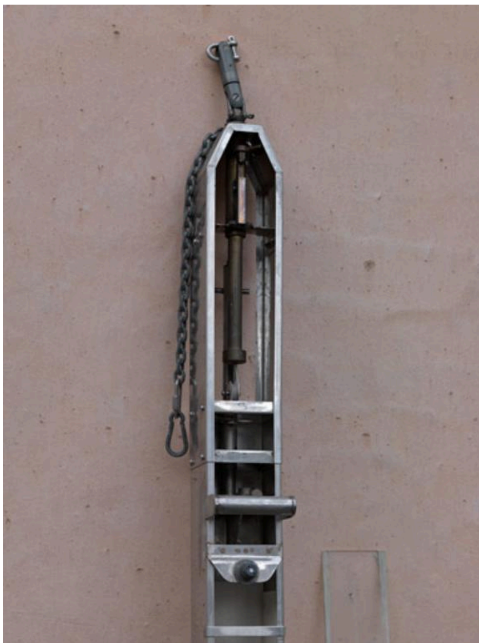
Carotier-main de 0,60m en bois (n'est plus utilisé)
