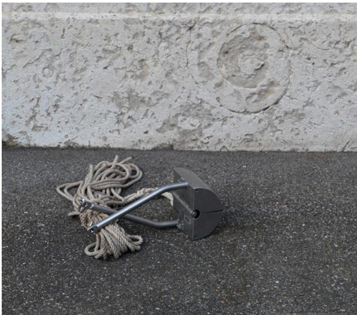
Benne type pince à sucre "Van Veen"
