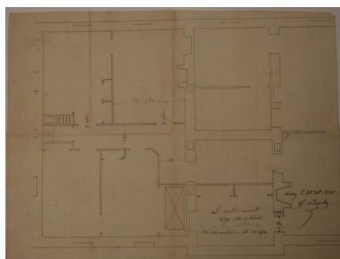
[Plan de l'étage (?) de la maison d'école d'Héry-sur-Alby]. Camille Ruphy, 25 oct 1880 5Héry-sur-Alby. Boîte Écoles). Phot. Thierry Monnet IVR84_20197400741NUCA
