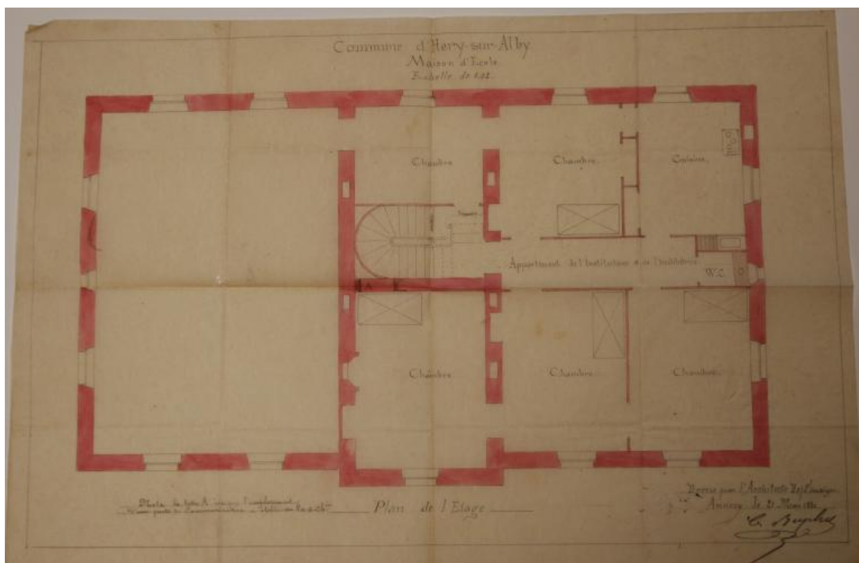
Maison d'École. Plan de l'Étage. Camille Ruphy, 21 mai 1880 (AC Héry-sur-Alby. Boîte Écoles).
