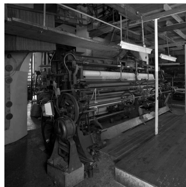
Métier à tisser (moteur Malécot St-
