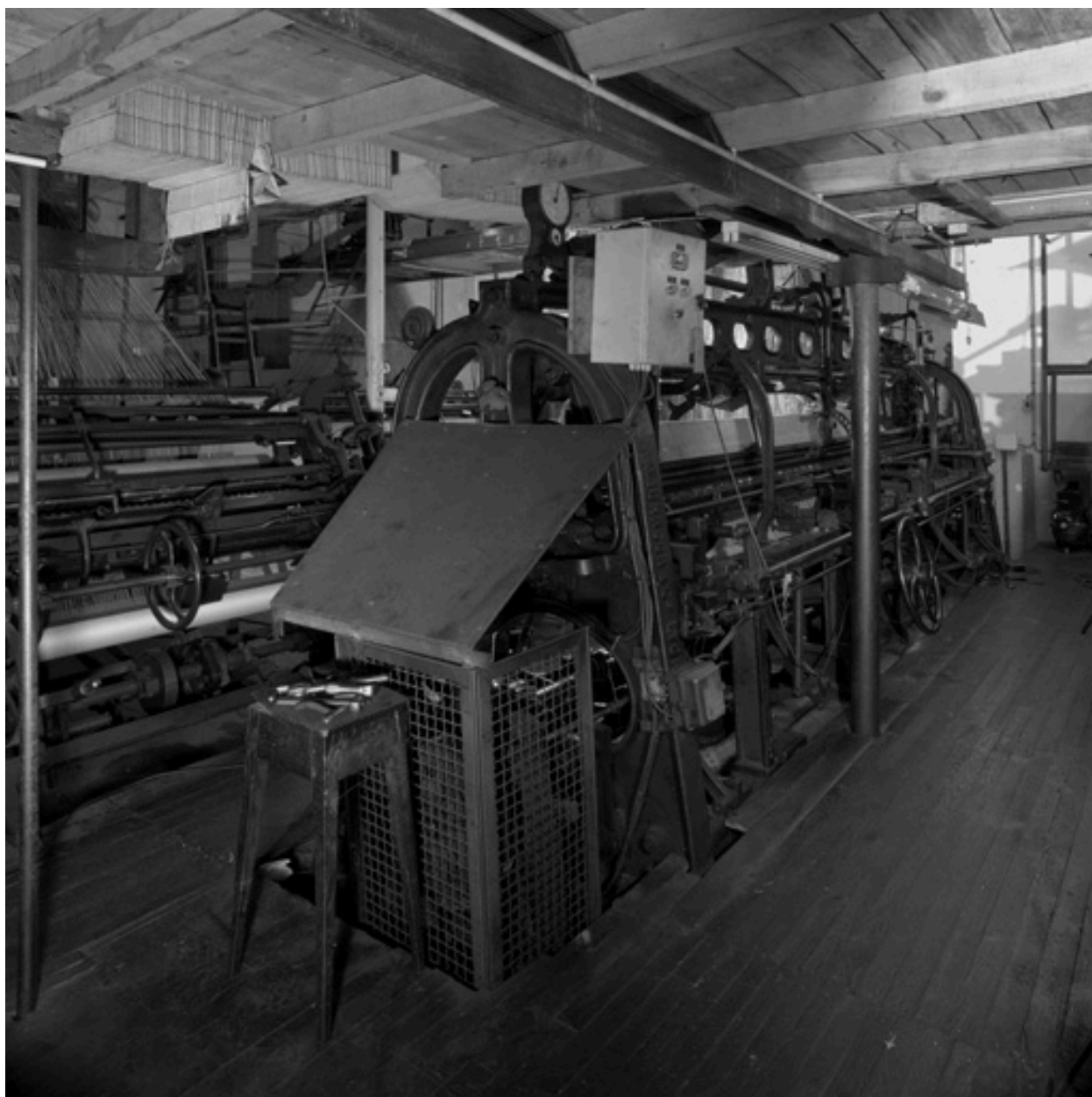
Métier à tisser la dentelle de marque Johnson 13,2 points, vue arrière
