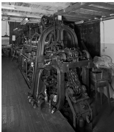
Métier à tisser de marque Johnson,
