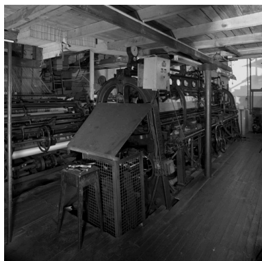
Métier à tisser la dentelle de marque
