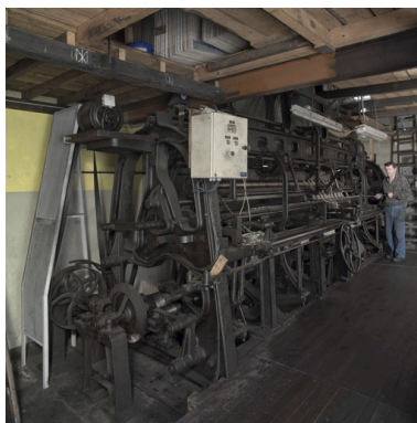
Métier dentelle : Johnson et Cie Lyon, (vue nord)
