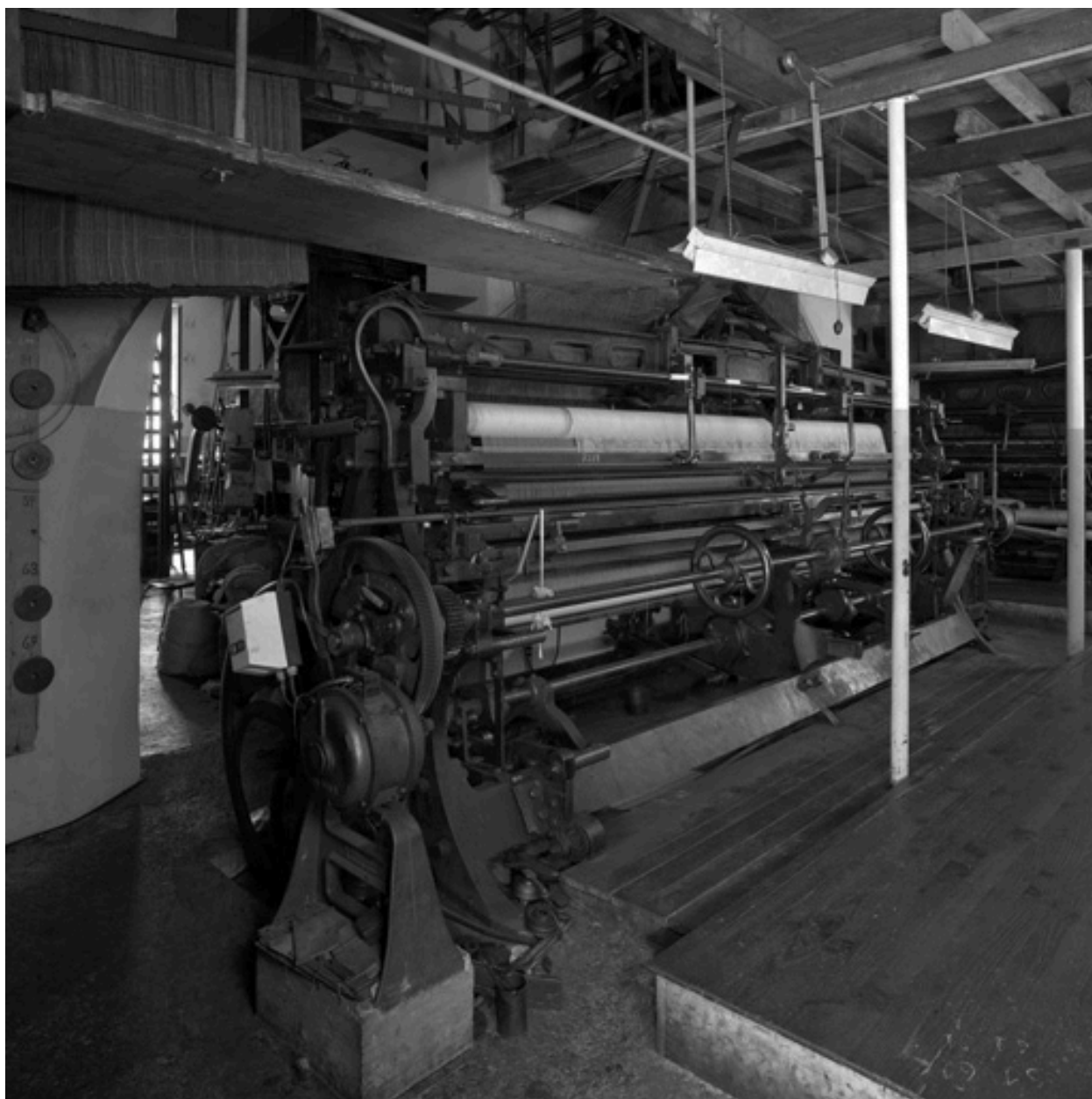
Métier à tisser (moteur Malécot St-Etienne), dit métier Bils 12,3 points
