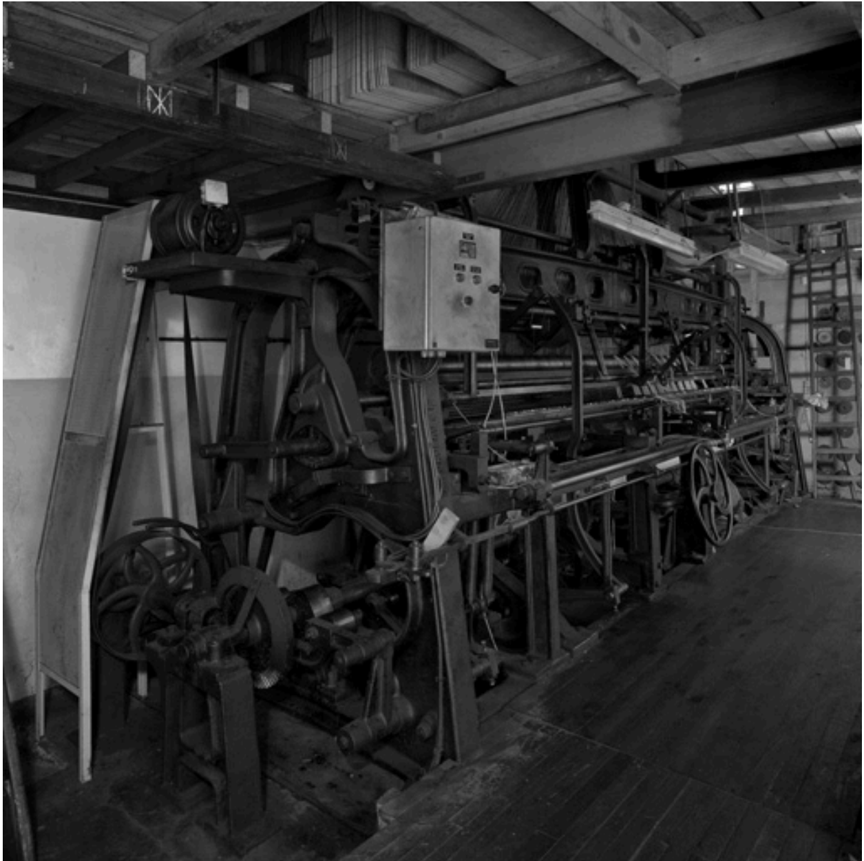
Métier dentelle : Johnson et Cie, vue nord
