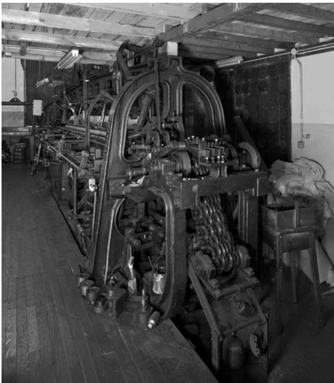
Métier à tisser de marque Johnson, détail latéral, chaîne d'entraînement
