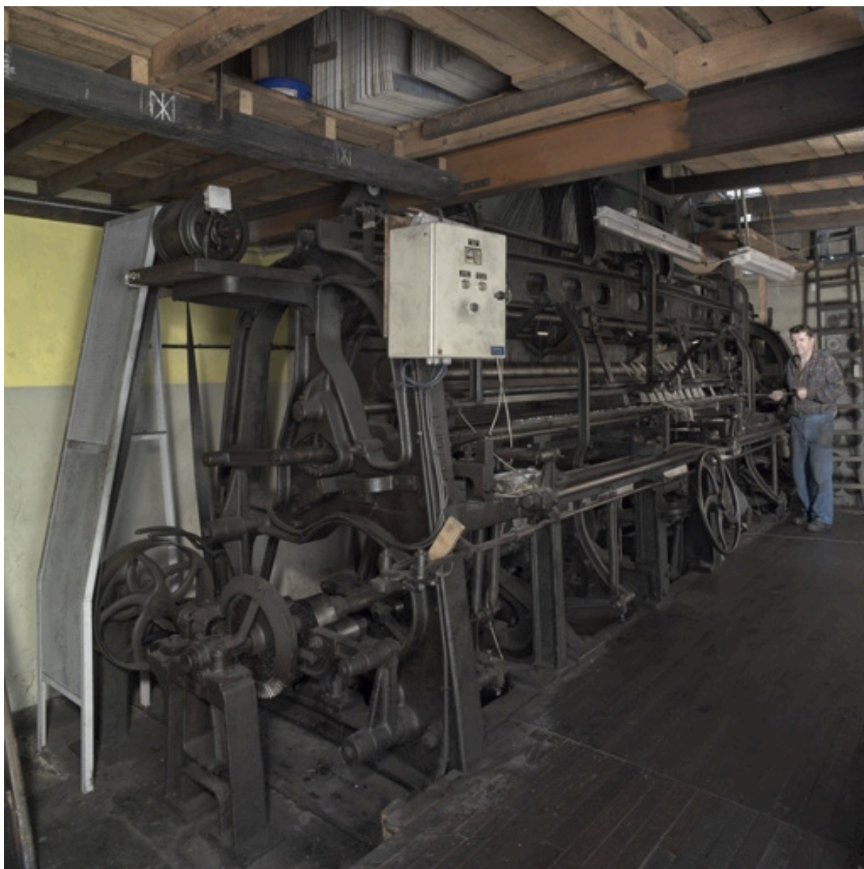
Métier dentelle : Johson et Cie Lyon, (vue nord)
