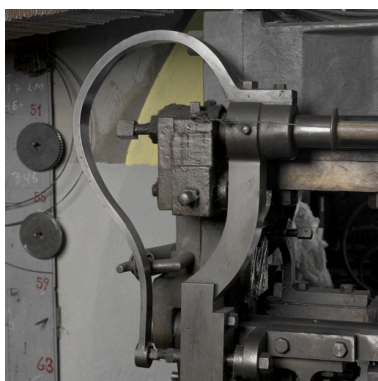
Détail métier Bils (moteur Malécot) Phot. Eric Dessert IVR82_20076901422NUCA
