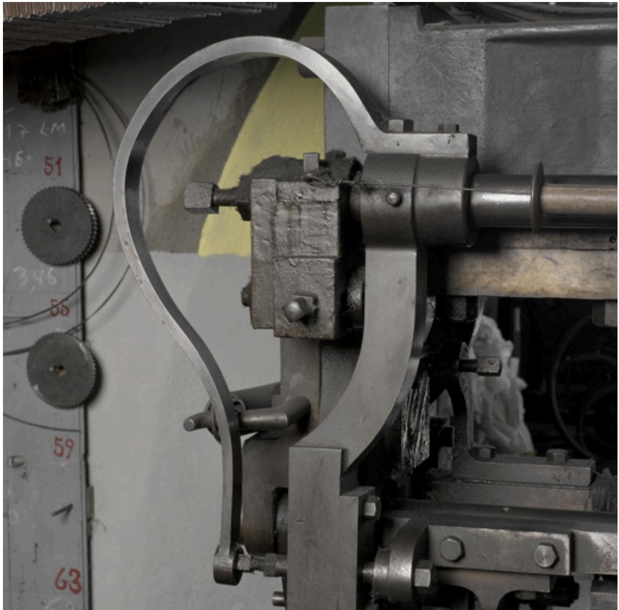
Détail métier Bils (moteur Malécot)
