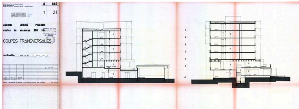
Accueil Loisirs Picardie. Coupes transversales / Atelier d'Architecture en Montagne, 10 février 1975 (AC Montricher-Albanne)
