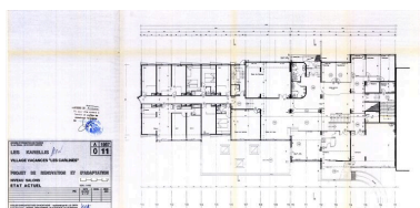
Village Vacances les Carlines. Projet de rénovation et d'adaptation. Plan niveau salon. Etat actuel / Atelier d'Architecture en Montagne, JG Orth, 6 octobre 1997 (AC Montricher-Albanne) Phot. Jean-François Lyon-Caen IVR82_20127302239NUC
