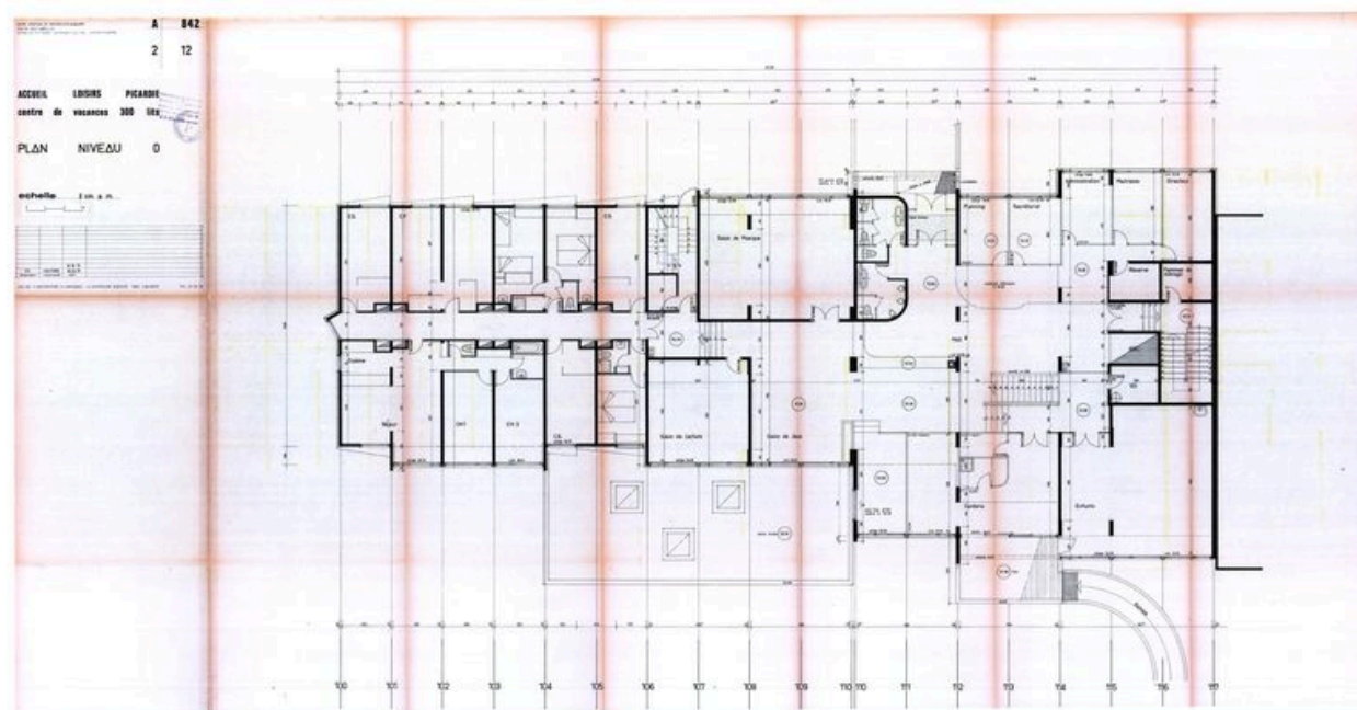
Accueil Loisirs Picardie. Plan niveau 0 / Atelier d'Architecture en Montagne, 29 avril 1975, rectifié 18 juin 1975 (AC Montricher-Albanne)
