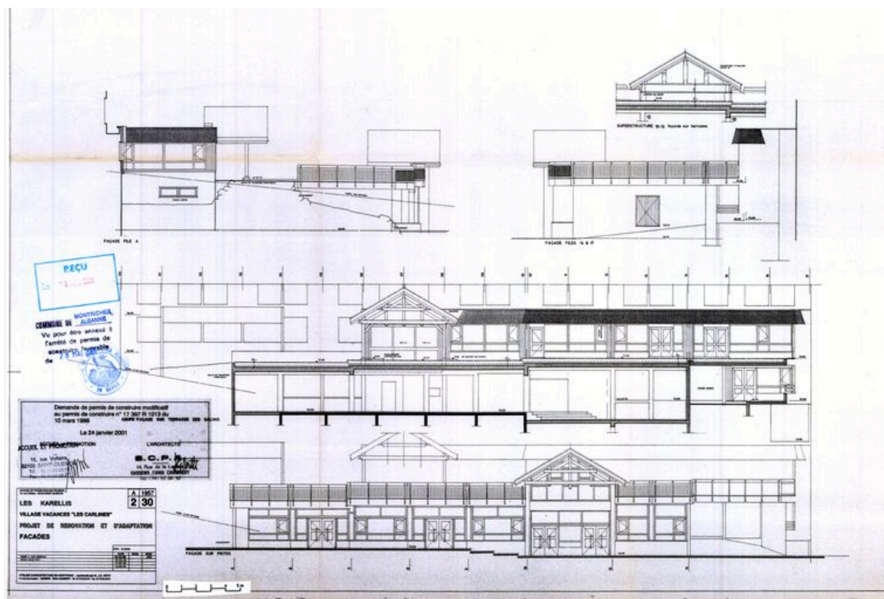
Village Vacances les Carlines. Projet de rénovation et d'adaptation. Elévations / Atelier d'Architecture en Montagne, JG Orth, 5 mars 1998. Remise à jour générale 25 février 2000 (AC Montricher-Albanne)
