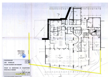
Village Vacances les Carlines. Projet de rénovation et d'adaptation. Plan niveau salle à manger / Atelier d'Architecture en Montagne, JG Orth, 6 octobre 1997 (AC Montricher-Albanne) Phot. Jean-François Lyon-Caen IVR82_20127302238NUC
