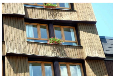
Détail de la structure de la façade et de l'essentage de planches Phot. Jean-François Lyon-Caen IVR82_20127302266NUCA
