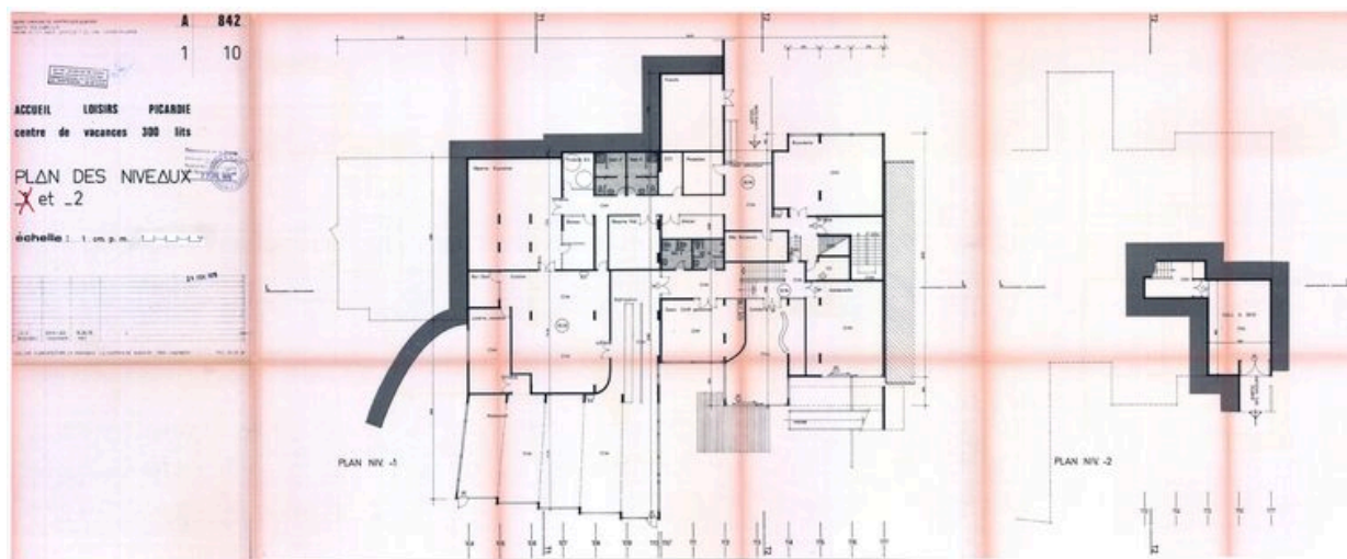
Accueil Loisirs Picardie. Plan niveau -2 / Atelier d'Architecture en Montagne, 10 février 1975 (AC Montricher-Albanne)
