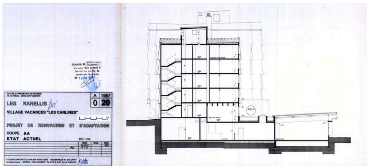
Village Vacances les Carlines. Projet de rénovation et d'adaptation. Coupe transversale. Etat actuel / Atelier d'Architecture en Montagne, JG Orth, 6 octobre 1997 (AC Montricher-Albanne)
