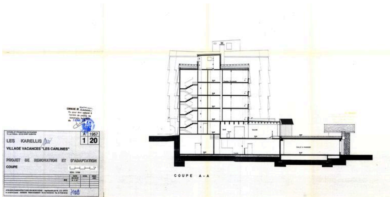
Village Vacances les Carlines. Projet de rénovation et d'adaptation. Coupe transversale / Atelier d'Architecture en Montagne, JG Orth, 6 octobre 1997 (AC Montricher-Albanne)
