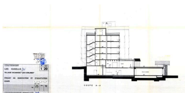
Village Vacances les Carlines. Projet de rénovation et d'adaptation. Coupe transversale / Atelier d'Architecture en Montagne, JG Orth, 6 octobre 1997 (AC Montricher-Albanne) Phot. Jean-François Lyon-Caen IVR82_20127302242NUC
