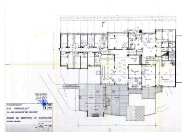
Village Vacances les Carlines. Projet de rénovation et d'adaptation. Plan niveau salon / Atelier d'Architecture en Montagne, JG Orth, 6 octobre 1997 (AC Montricher-Albanne) Phot. Jean-François Lyon-Caen IVR82_20127302240NUC
