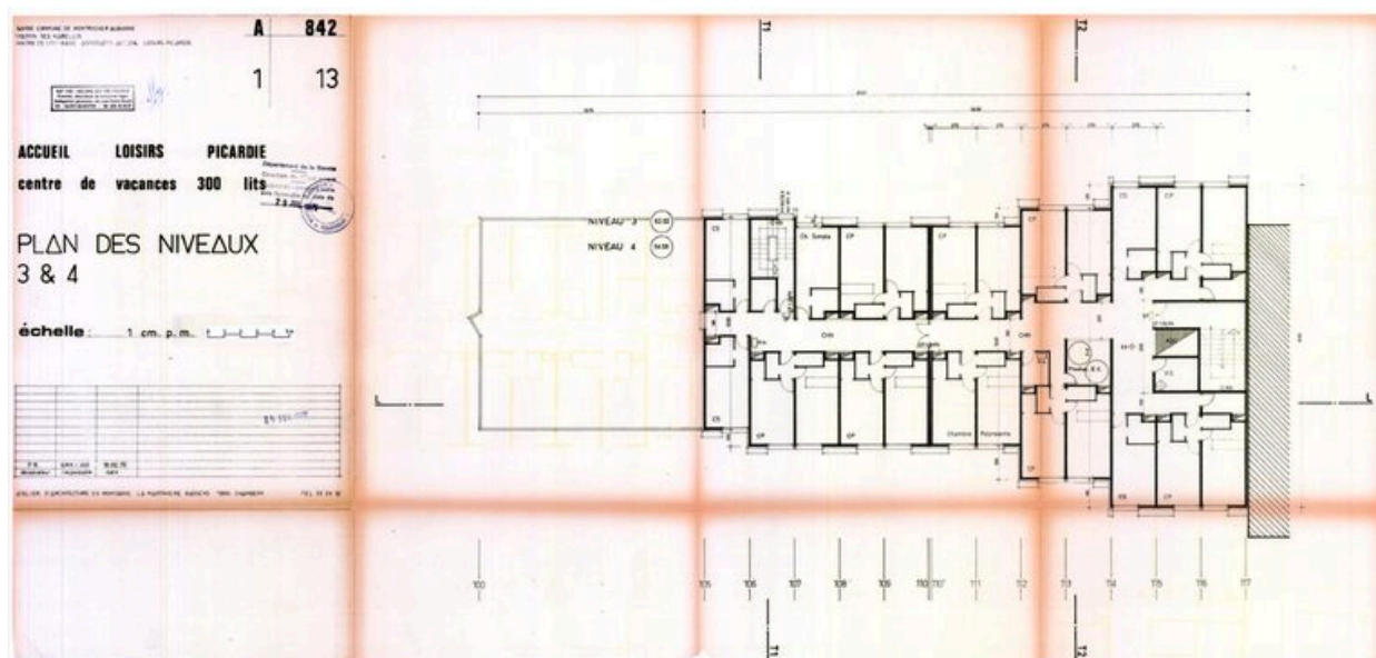
Accueil Loisirs Picardie. Plan niveau 3 et 4 / Atelier d'Architecture en Montagne, 10 février 1975 (AC Montricher-Albanne)
