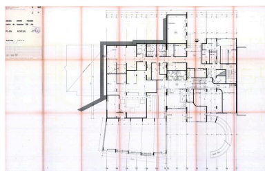
Accueil Loisirs Picardie. Plan niveau -1 / Atelier d'Architecture en Montagne, 29 avril 1975, rectifié 18 juin 1975 (AC Montricher-Albanne) Phot. Jean-François Lyon-Caen IVR82_20127302203NUC
