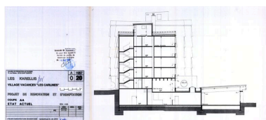
Village Vacances les Carlines. Projet de rénovation et d'adaptation. Coupe transversale. Etat actuel / Atelier d'Architecture en Montagne, JG Orth, 6 octobre 1997 (AC Montricher-Albanne) Phot. Jean-François Lyon-Caen IVR82_20127302241NUC
