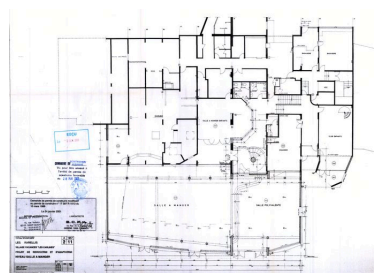
Village Vacances les Carlines. Projet de rénovation et d'adaptation. Niveau salle à manger / Atelier d'Architecture en Montagne,
