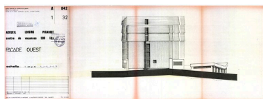
ACCueil Loisirs Picardie. Elévation ouest / Atelier d'Architecture en Montagne, 10 février 1975, rectifié 11 juin 1975 (AC Montricher-Albanne) Phot. Jean-François Lyon-Caen IVR82_20127302212NUC
