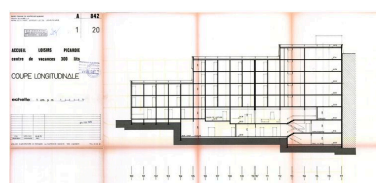
Accueil Loisirs Picardie. Coupe longitudinale / Atelier d'Architecture en Montagne, 10 février 1975 (AC Montricher-Albanne) Phot. Jean-François Lyon-Caen IVR82_20127302208NUC
