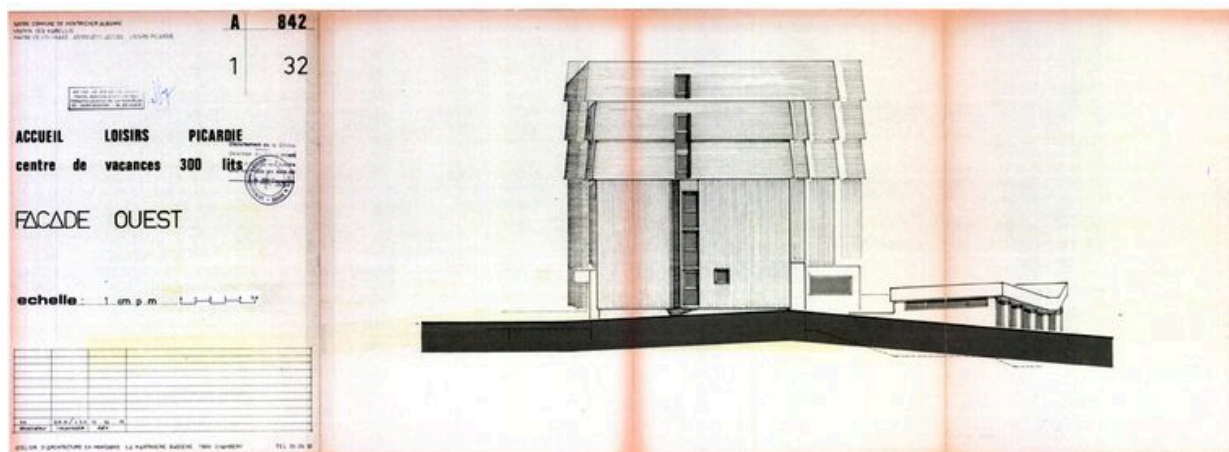
ACCueil Loisirs Picardie. Elévation ouest / Atelier d'Architecture en Montagne, 10 février 1975, rectifié 11 juin 1975 (AC Montricher-Albanne)
