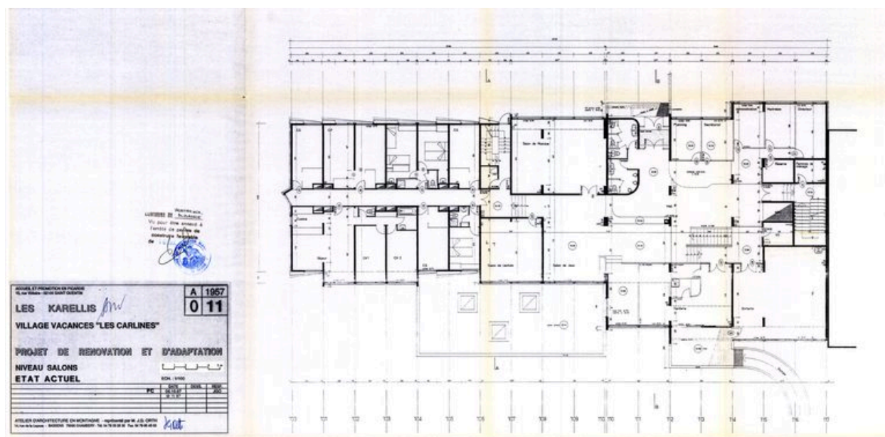
Village Vacances les Carlines. Projet de rénovation et d'adaptation. Plan niveau salon. Etat actuel / Atelier d'Architecture en Montagne, JG Orth, 6 octobre 1997 (AC Montricher-Albanne)
