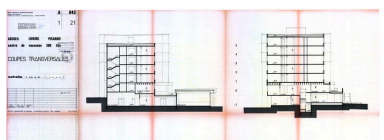
Accueil Loisirs Picardie. Coupes transversales / Atelier d'Architecture en Montagne, 10 février 1975 (AC Montricher-Albanne) Phot. Jean-François Lyon-Caen IVR82_20127302209NUC
