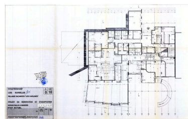
Village Vacances les Carlines. Projet de rénovation et d'adaptation. Plan niveau salle à manger. Etat actuel / Atelier d'Architecture en Montagne, JG Orth, 6 octobre 1997 (AC Montricher-Albanne) Phot. Jean-François Lyon-Caen IVR82_20127302237NUC
