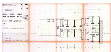
Accueil Loisirs Picardie. Plan niveau 3 et 4 / Atelier d'Architecture en Montagne, 10 février 1975 (AC Montricher-Albanne) Phot. Jean-François Lyon-Caen IVR82_20127302206NUC
