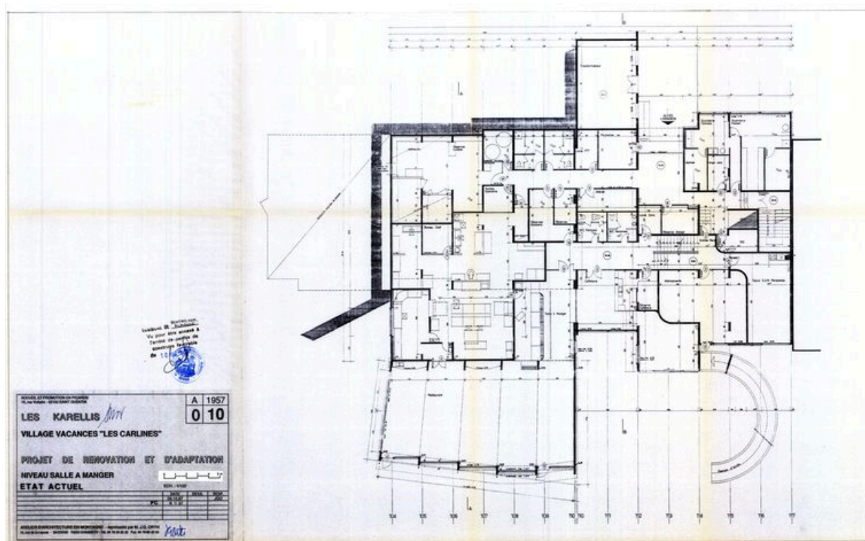
Village Vacances les Carlines. Projet de rénovation et d'adaptation. Plan niveau salle à manger. Etat actuel / Atelier d'Architecture en Montagne, JG Orth, 6 octobre 1997 (AC Montricher-Albanne)
