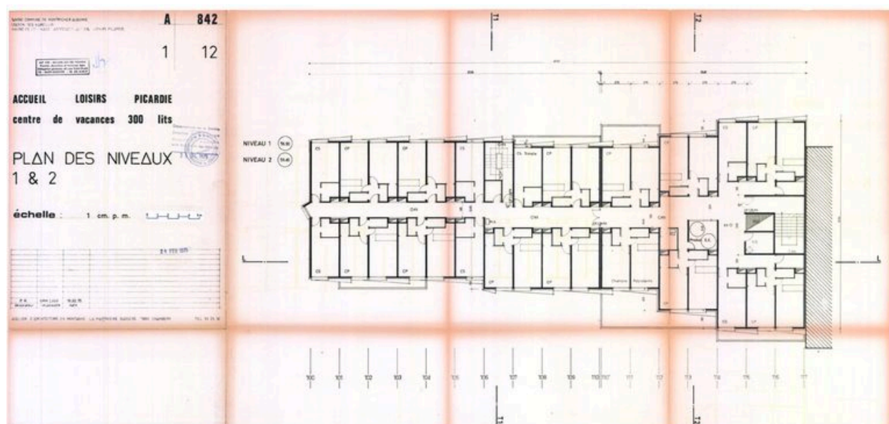
Accueil Loisirs Picardie. Plan niveaux 1 et 2 / Atelier d'Architecture en Montagne, 10 février 1975 (AC Montricher-Albanne)
