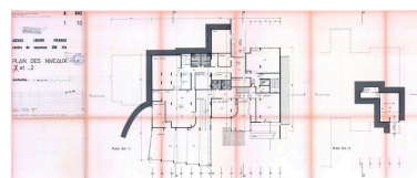
Accueil Loisirs Picardie. Plan niveau -2 / Atelier d'Architecture en Montagne, 10 février 1975 (AC Montricher-Albanne) Phot. Jean-François Lyon-Caen IVR82_20127302202NUC
