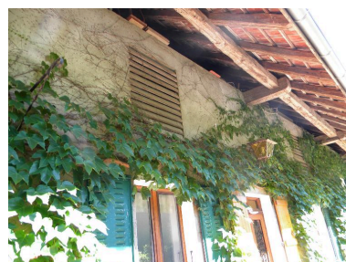
Vue des poutres solives sous le débord de toit (2008 F4 603). Phot. Jérôme Daviet IVR82_20137401117NUCA
