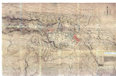
Master plan for a new mountain town in the Hte Savoie. Plan masse. M. Breuer, L. Chappis, A. Gaillard, Atelier d'Architecture à Courchevel, G. Chervaz architectes, 31 mars 1961. Révisé en 1961 et le 2 avril 1962 (AC Arâches-la-Frasse) Phot. Jean-François Lyon-Caen, Phot. C. Salomon-Pelen, Autr. Breuer Marcel (architecte), Autr. Laurent Chappis, Autr. Gaillard André (architecte), Autr. Chervaz Gérard (architecte) IVR82_20127401471NUCA
