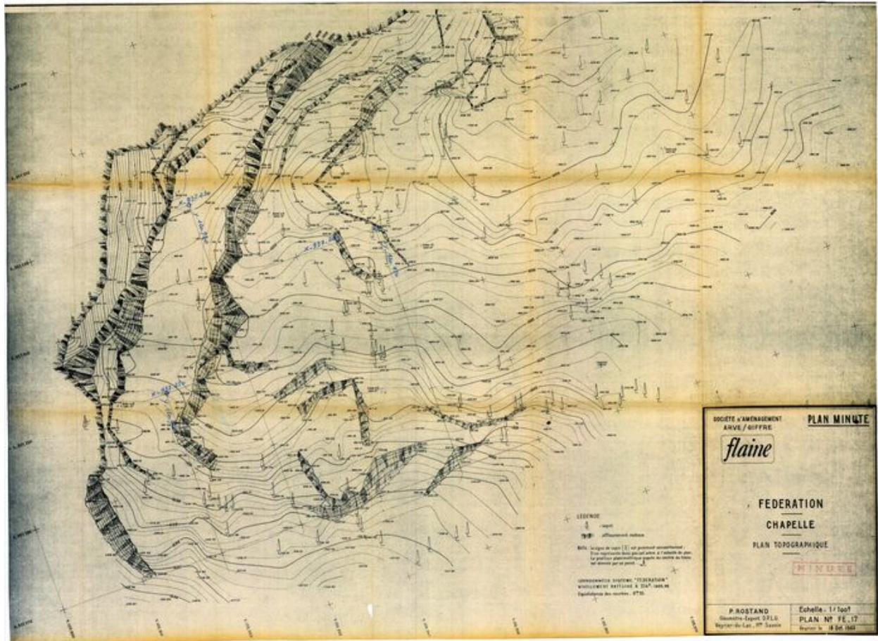
Fédération. Chapelle. Plan topographique. P. Rostang, géomètre expert, 13 octobre 1963. Modification A, 31 décembre 1963 : extension de la zone sud. Détail (AC Arâches-la Frasse)
