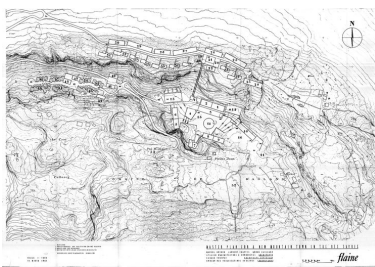
Master plan for a new mountain town in the Hte Savoie. Marcel Breuer, Laurent Chappis, André Gaillard, Atelier d'Architecture à Courchevel, Gérard Chervaz architecte assistant, 14 mars 1961 (AC Arâches-la-Frasse). Phot. Jean-François Lyon-Caen, Phot. C. Salomon-Pelen, Autr. Breuer Marcel (architecte), Autr. Laurent Chappis, Autr. Gaillard André (architecte), Autr. Chervaz Gérard (architecte) IVR82_20127401463NUC
