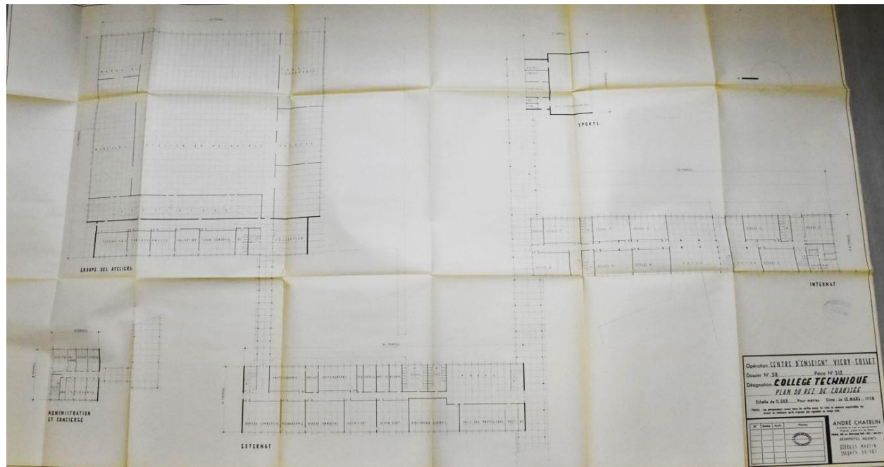
Centre d'enseignement. Partie collège technique. Plan du rez-de-chaussée, par A. Chatelin, G. martin, J. Brière, 7 mars 1958 (AC Vichy. 13 W 5).
