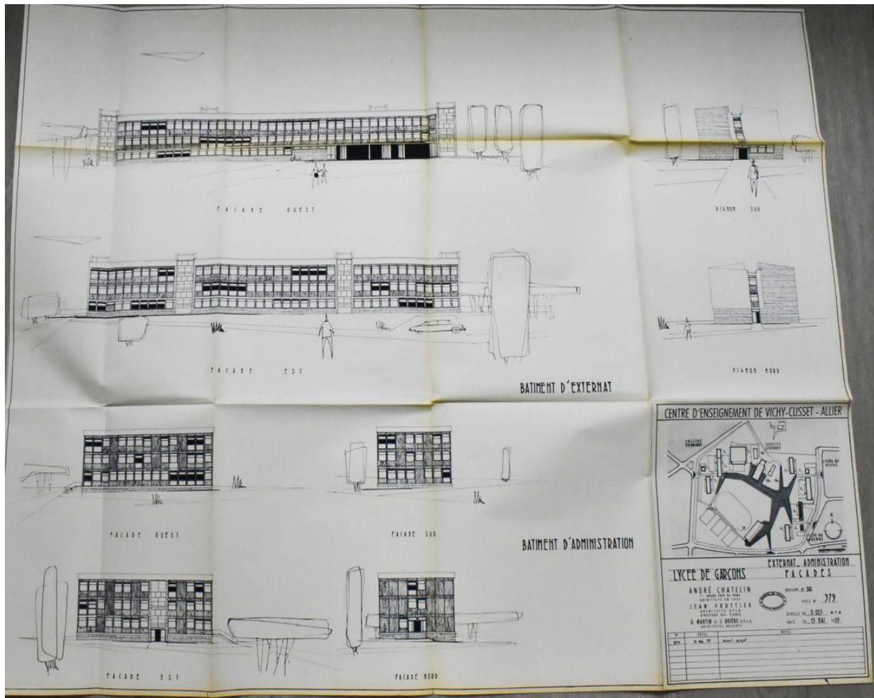
Centre d'enseignement Vichy-Cusset. Lycée de garçons. Externat et administration. Façades, par A. Chatelin, G. martin, J. Brière, 7 mars 1958 (AC Vichy. 13 W 5).
