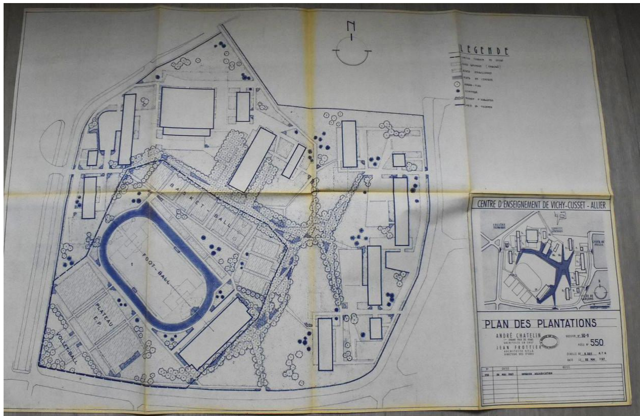
Centre d'enseignement Vichy-Cusset. Dossier d'adjudication. Plan des plantations, par A. Chatelin, J. Frottier, 20 mai 1961 (AC Vichy. 13 W 6).
