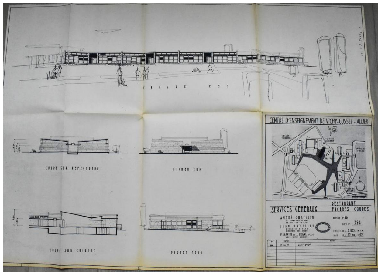
Centre d'enseignement Vichy-Cusset. Services généraux, restaurant. Façades et coupes, par A. Chatelin, J. Frottier, G. Martin, J. Brière, 15 mai 1959 (AC Vichy. 13 W 5). (AC Vichy. 13 W 5).
