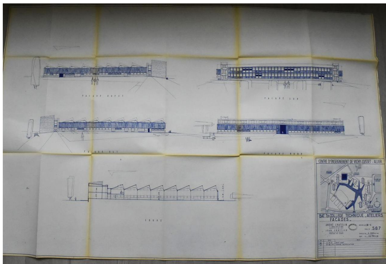
Centre d'enseignement Vichy-Cusset. Dossier d'adjudication. Bâtiment T5 (collège technique : ateliers). Façades, par A. Chatelin, J. Frottier, 20 mai 1961 (AC Vichy. 13 W 6).
