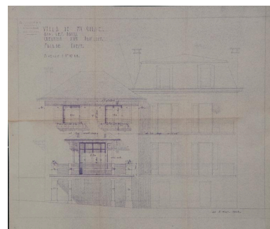
Façade ouest, 1943 Repro. Denys Harreau IVR82_20137301054NUCB
