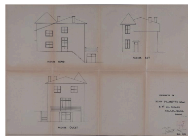
Agrandissement : élévations, 1972 Repro. Denys Harreau IVR82_20157301111NUCB
