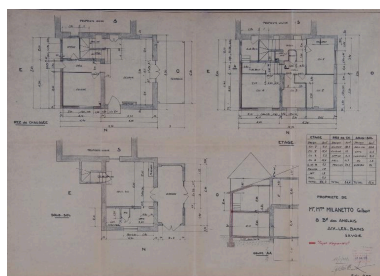
Agrandissement : plans et coupe, 1972 Repro. Denys Harreau
