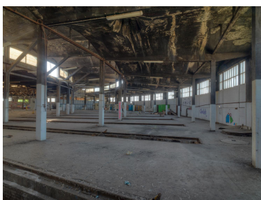
Vue d'ensemble latéral des fosses de réparation Phot. Martial Couderette IVR82_20156901718NUCAQ
