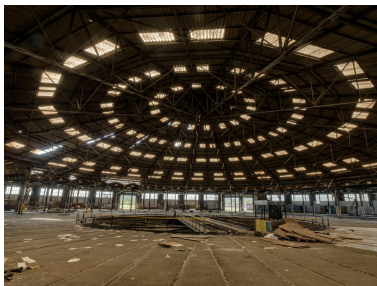
Vue intérieur de la rotonde de grigny Phot. Martial Couderette IVR82_20156901701NUCAQ
