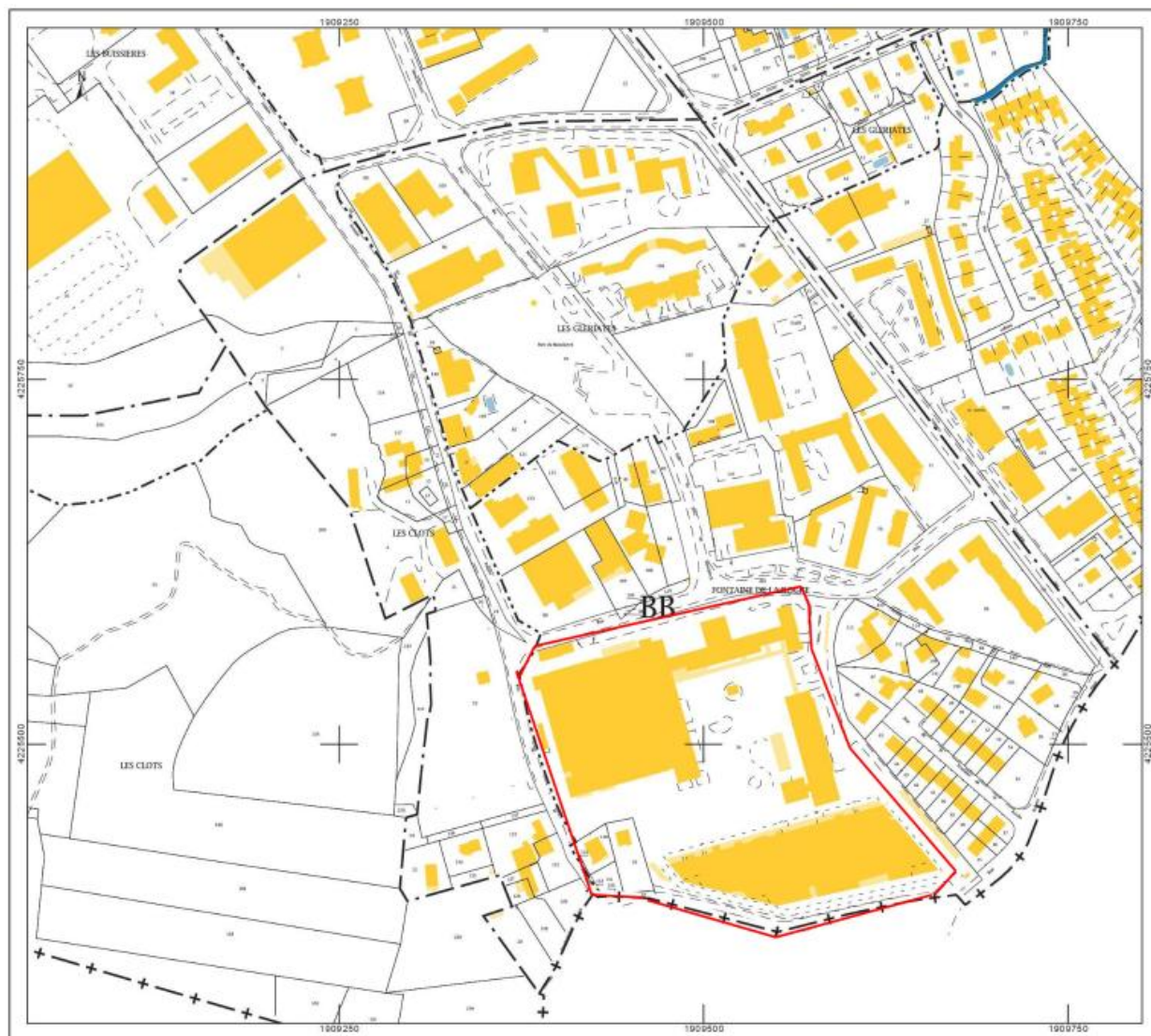
Plan masse et de situation, extrait du plan cadastral
