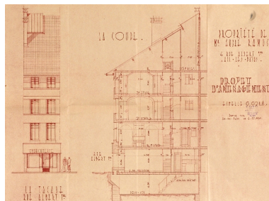
Coupe et élévation Repro. François Fouger IVR82_20057302011NUCB
