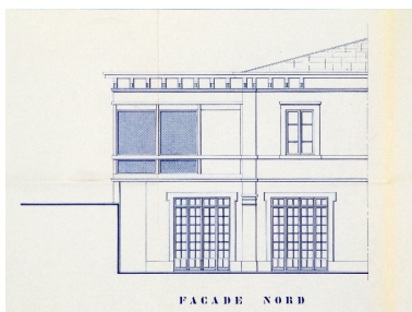
Elévation nord de l'extension Repr. François Fouger IVR82_20097300008NUCB
