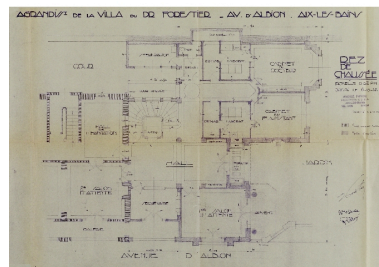
Plan du rez-de-chaussée Repr. François Fouger IVR82_20097300013NUCB
