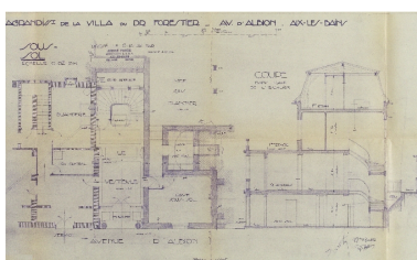
Plan du sous-sol Repr. François Fouger IVR82_20097300012NUCB
