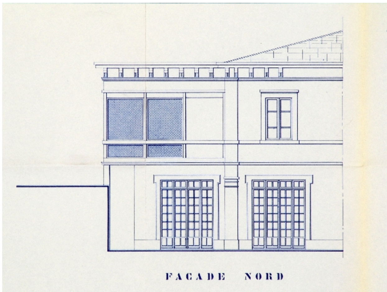
Elévation nord de l'extension
