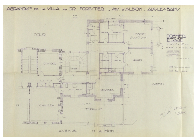
Plan du 1er étage Repr. François Fouger IVR82_20097300014NUCB
