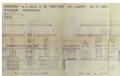
Elévations ouest et sud Repr. François Fouger IVR82_20097300011NUCB
