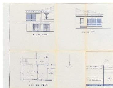
Plan et élévations de l'extension Repr. François Fouger IVR82_20097300007NUCB
