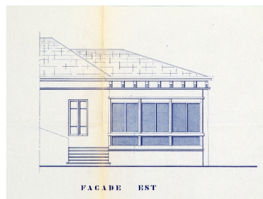
Elévation est de l'extension Repr. François Fouger IVR82_20097300009NUCB
