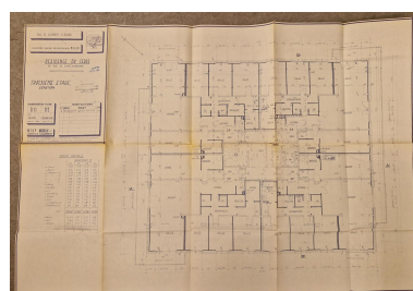
Plan du 3e étage de la résidence. Repro. Brigitte Ceroni, Autr. auteur inconnu IVR84_20256301424NUCA
