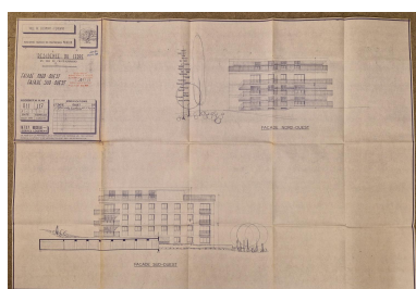
Elévations nord-ouest et sud-ouest de l'immeuble. Repro. Brigitte Ceroni, Autr. auteur inconnu IVR84_20256301428NUCA
