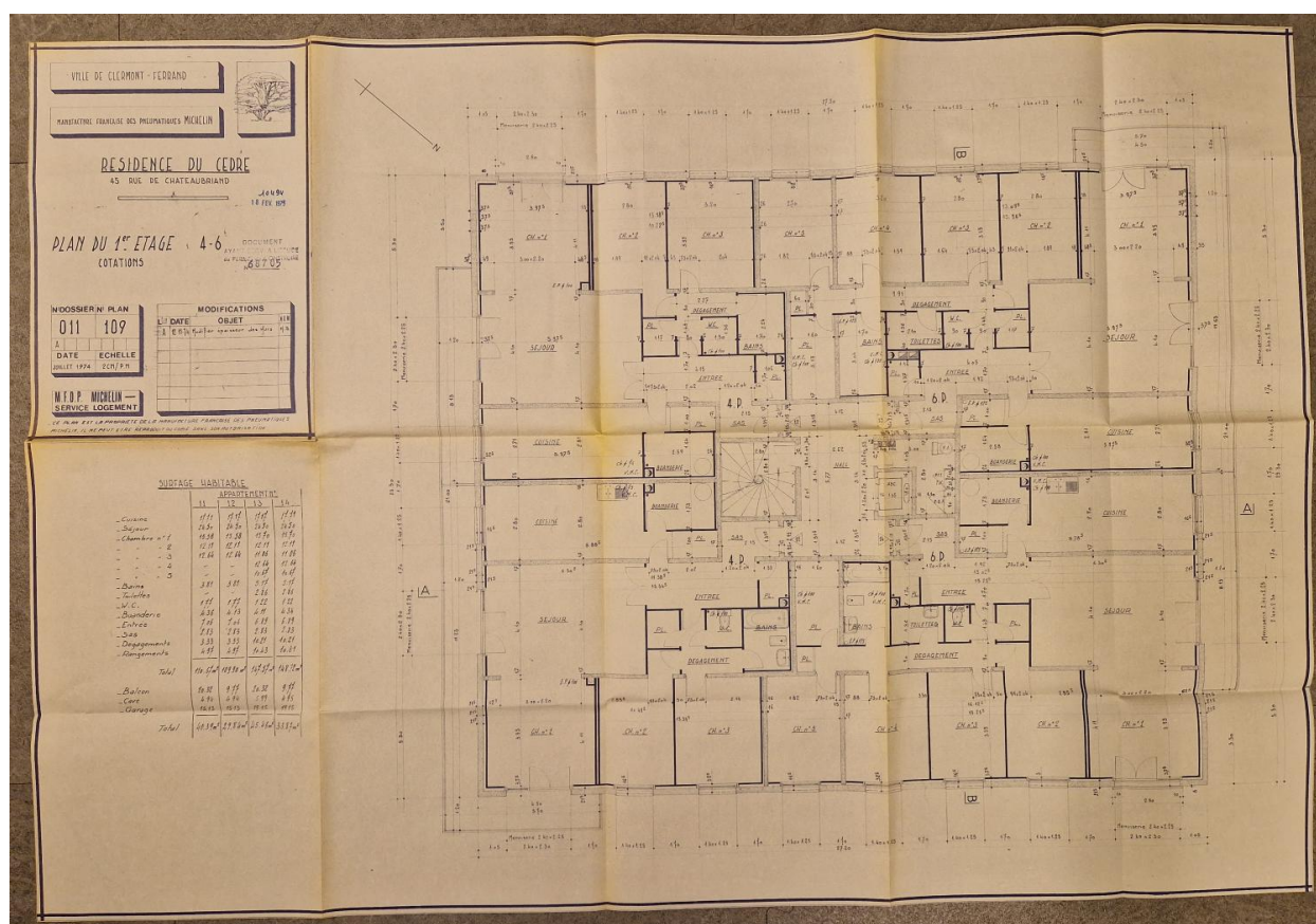
Plan du 1er étage de la résidence.
