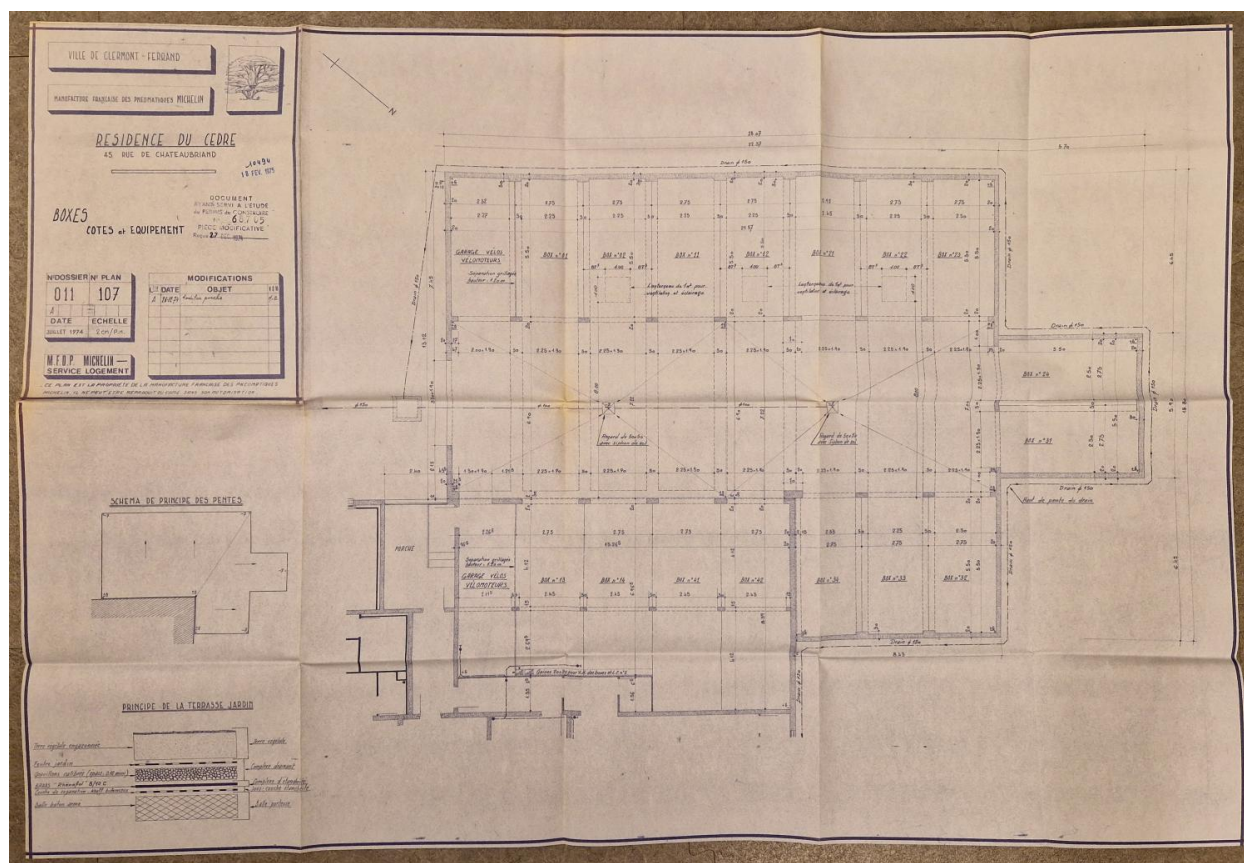
Plan des boxes et du garage à vélos de la résidence.
