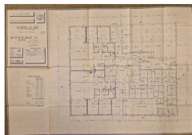
Plan du rez-de- chaussée de la résidence. Repro. Brigitte Ceroni, Autr. auteur inconnu IVR84_20256301421NUCA
