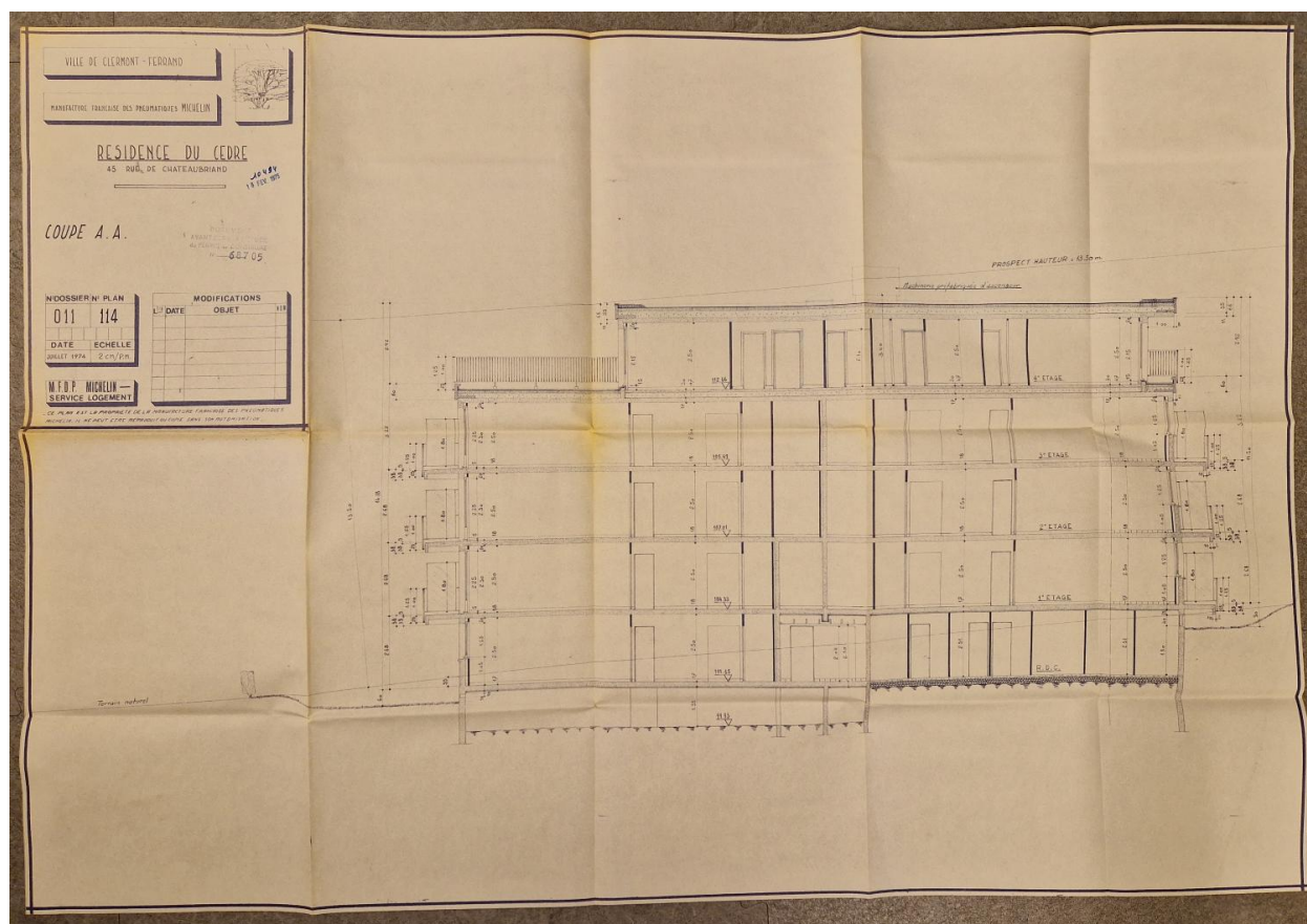
Coupe AA de l'immeuble.
