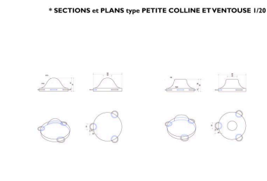
Sections et plans type Petite colline et Ventouse 1/20. Autr. Polly Brotherhood, Autr. Julia Maendler IVR84_20204200110NUDA
