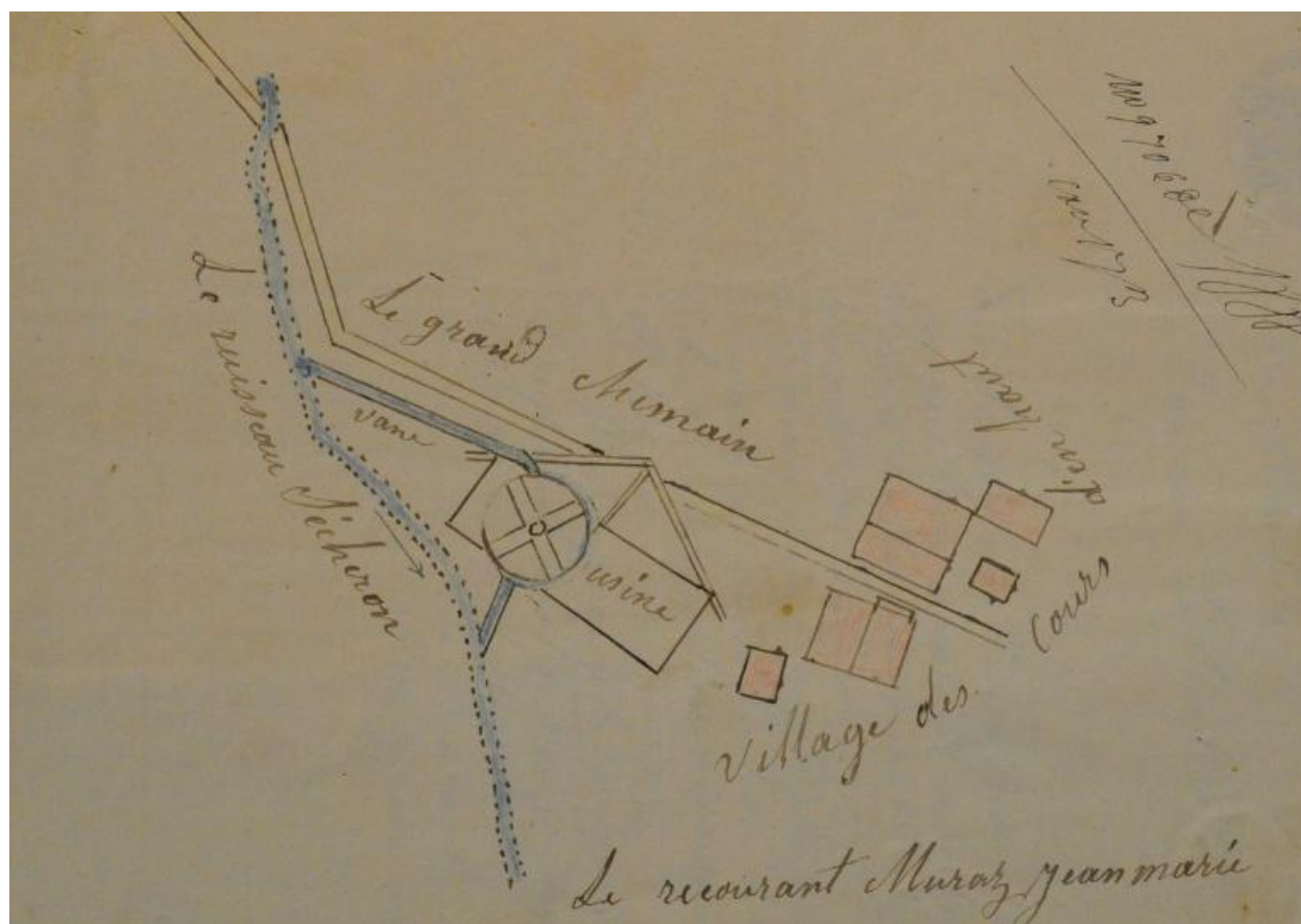
Plan de la scierie, 1888 (FR.AD073, 83S8).
