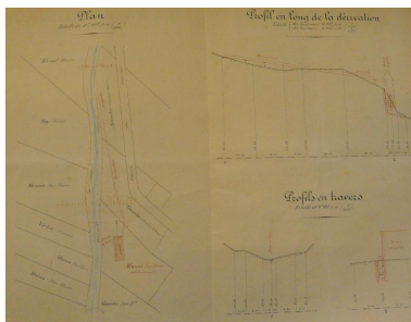
Plan de la scierie, 1888 (FR.AD073, 83S8). IVR84_20167302620NUCA
