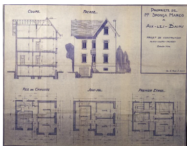
Plans, coupe et élévation, 1931 Repro. Denys Harreau IVR84_20177300260NUCB
