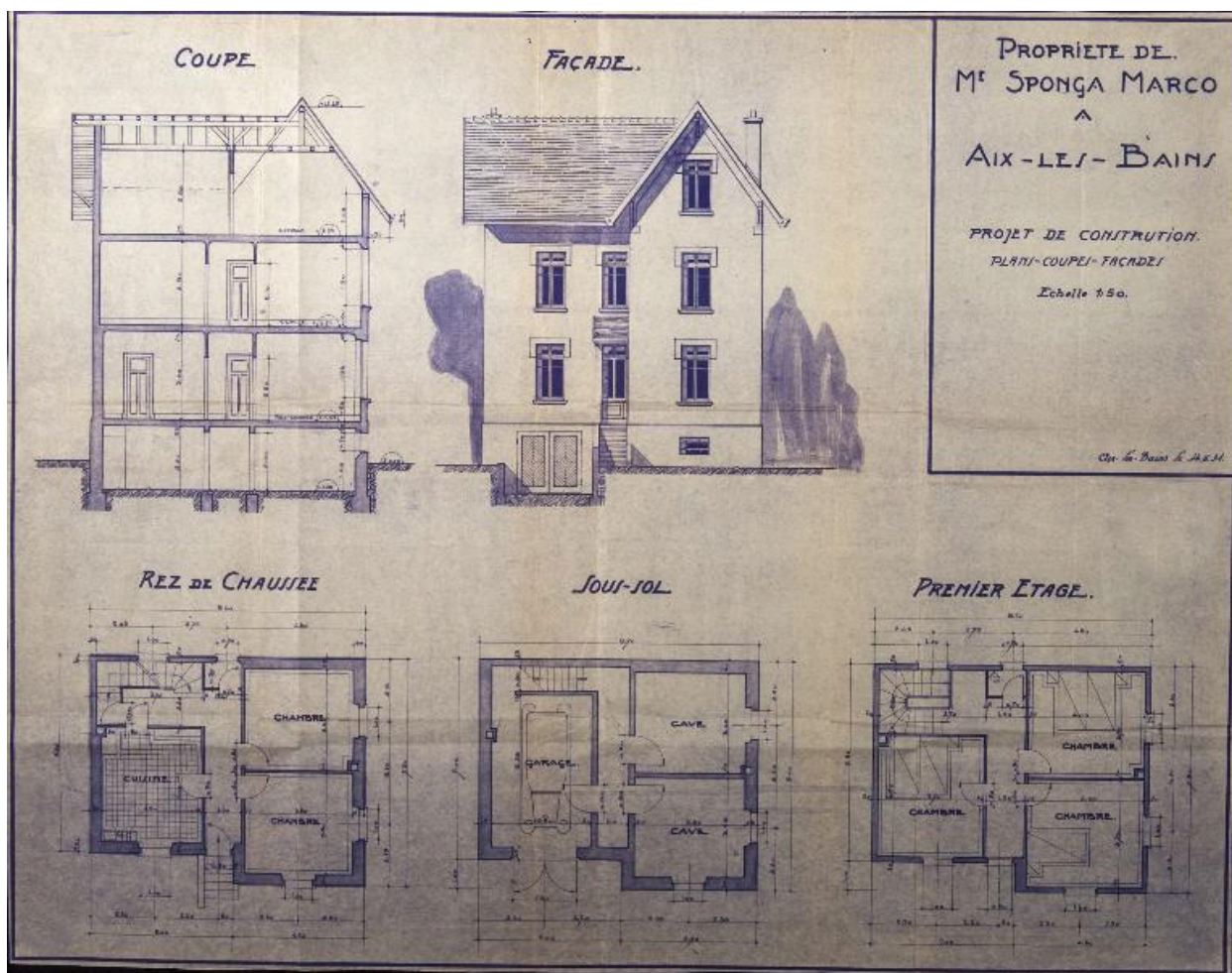
Plans, coupe et élévation, 1931
