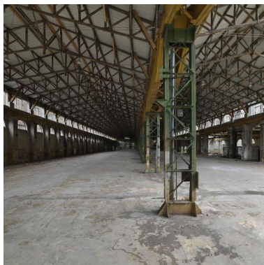
Vue du grand système de charpente en bois des halles de Couzon.
