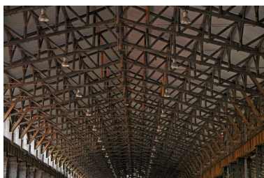
Détail charpente en bois
