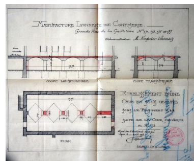
Plan du sous-sol, par François Clermont, 1913 (AC Lyon) Phot. Catherine Guégan IVR84_20166901837NUCA
