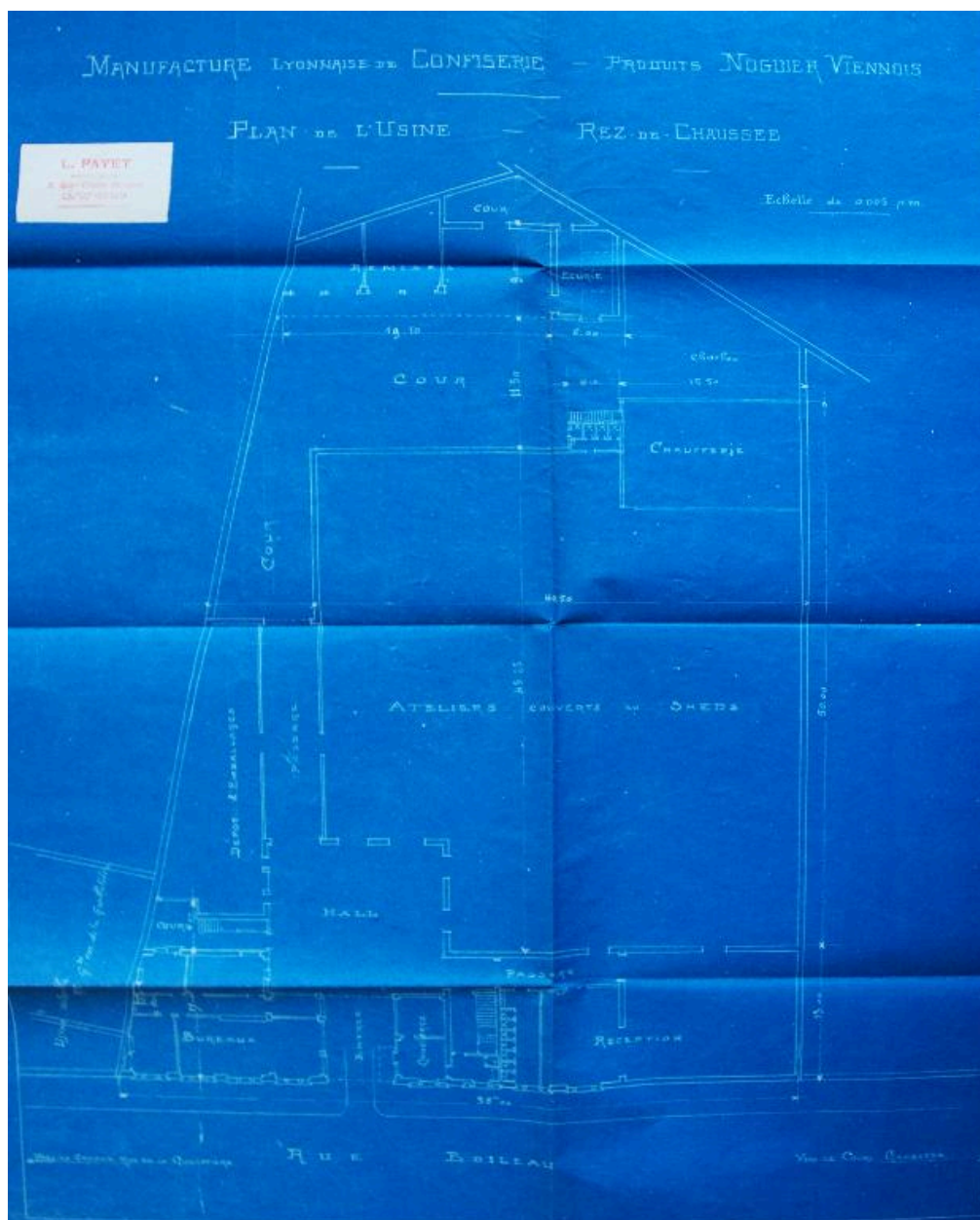
Plan du rez-de-chaussée de l'usine, par Louis Payet (AC Lyon)
