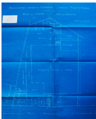
Plan du rez-de-chaussée de l'usine, par Louis Payet (AC Lyon) Phot. Catherine Guégan IVR84_20166901833NUCA
