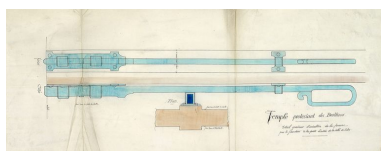
Dessin technique d'exécution de la ferrure pour la fermeture de la porte de la salle de culte. Repro. Didier Gourbin, Autr. Gaspard André IVR82_20106906126NUCA
