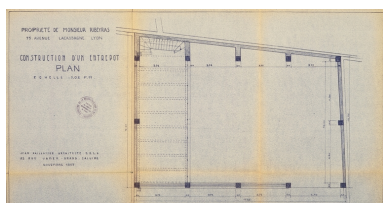
AC Lyon : 354 WP 068 PCA n° 687, plan du hangar pour M. Ribeyras par M. Paillason, 1957 Repro. Gilles Bernasconi IVR82_20096901865NUCA
