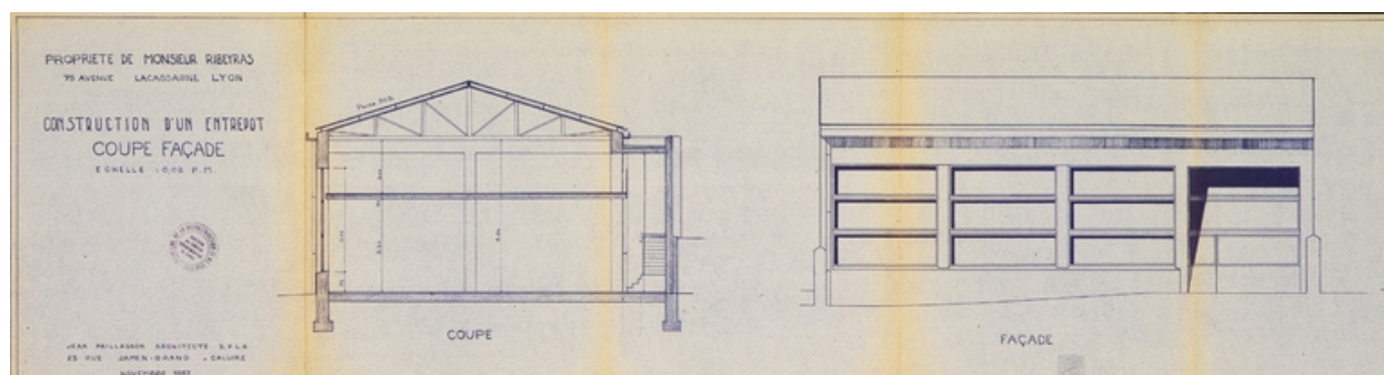
AC Lyon : 354 WP 068 PCA n° 687, façade et coupe du hangar pour M. Ribeyras par M. Paillason, 1957
