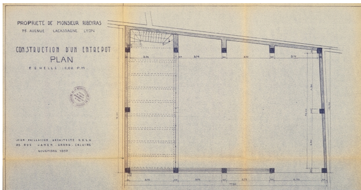
AC Lyon : 354 WP 068 PCA n° 687, plan du hangar pour M. Ribeyras par M. Paillason, 1957
