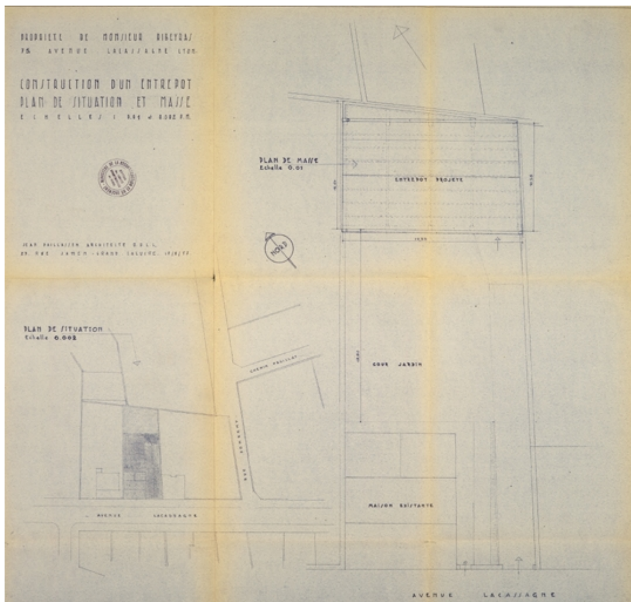
AC Lyon : 354 WP 068 PCA n° 687, plan de situation et plan masse du hangar pour M. Ribeyras par M. Paillason, 1957
