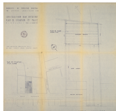
AC Lyon : 354 WP 068 PCA n° 687, plan de situation et plan masse du hangar pour M. Ribeyras par M. Paillason, 1957 Repro. Gilles Bernasconi IVR82_20096901864NUCA
