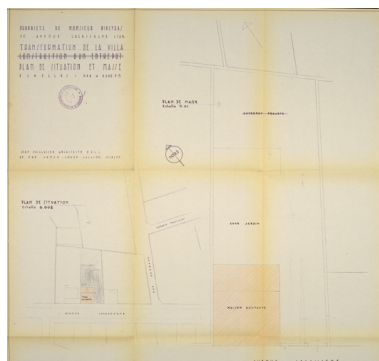
AC Lyon : 354 WP 056 PCA n° 556, plan de situation, entrepôt et villa de monsieur Ribeyras 1957. Repro. Gilles Bernasconi IVR82_20096901862NUCA
