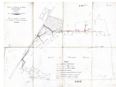
Plan de la base aérienne de Lyon-Bron vers 1926 (ADR : 4535W47) Phot. Nadine Halitim-Dubois IVR84_20256900112NUC
