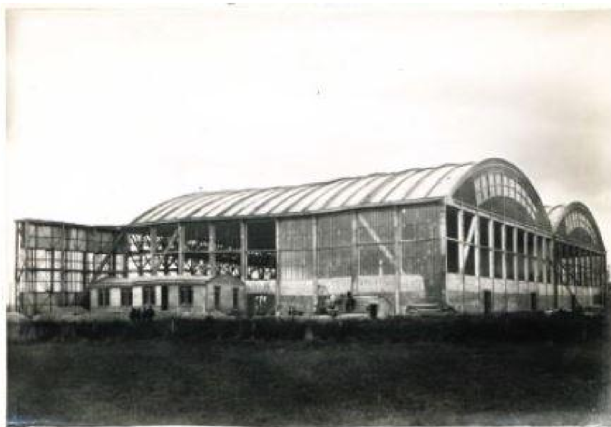
Hangar VI photo chantier ETs. Boussiron 1925 (ADR : 4535W47)
