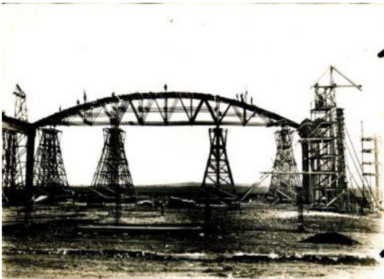
Hangar VI photo chantier ETs. Boussiron (ADR 1925 : 4535W47)
