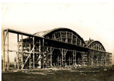
Hangar VI photo chantier ETs. Boussiron en 1925 (ADR : 4535W47) Phot. Nadine Halitim-Dubois IVR84_20256900102NUC
