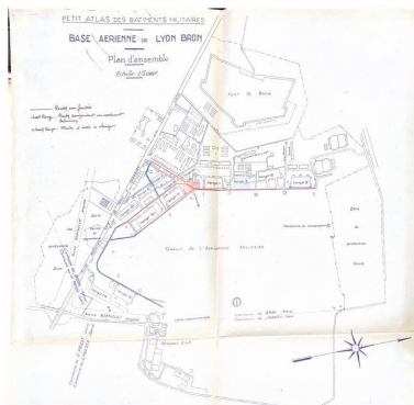
Plan de la base aérienne de Lyon-Bron vers 1926 (ADR : 4535W47) Phot. Nadine Halitim-Dubois IVR84_20256900110NUCA
