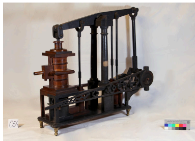
Machine à vapeur, vue de côté Phot. Krystelle Besson , Phot. Mirco Meier, Phot. Marion Petit IVR84_20256901074NUCA
