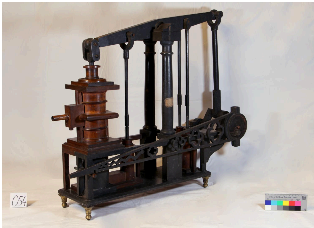
Machine à vapeur, vue de côté
