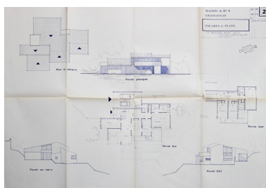
Châteaugay, la Maison R., plans des niveaux bas et haut, façades sud, est et ouest, François-Yves BERNARD architecte, 1975 (Archives municipales de Châteaugay). Repro. Christophe Laurent, Autr. François-Yves Bernard IVR84_20216302428NUCA
