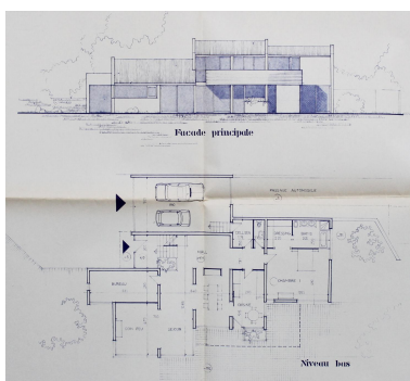
Châteaugay, la Maison R., plan du niveau bas et façade principale (sud), François-Yves BERNARD architecte, 1975 (Archives municipales de Châteaugay). Repro. Christophe Laurent, Autr. François-Yves Bernard IVR84_20216302429NUCA
