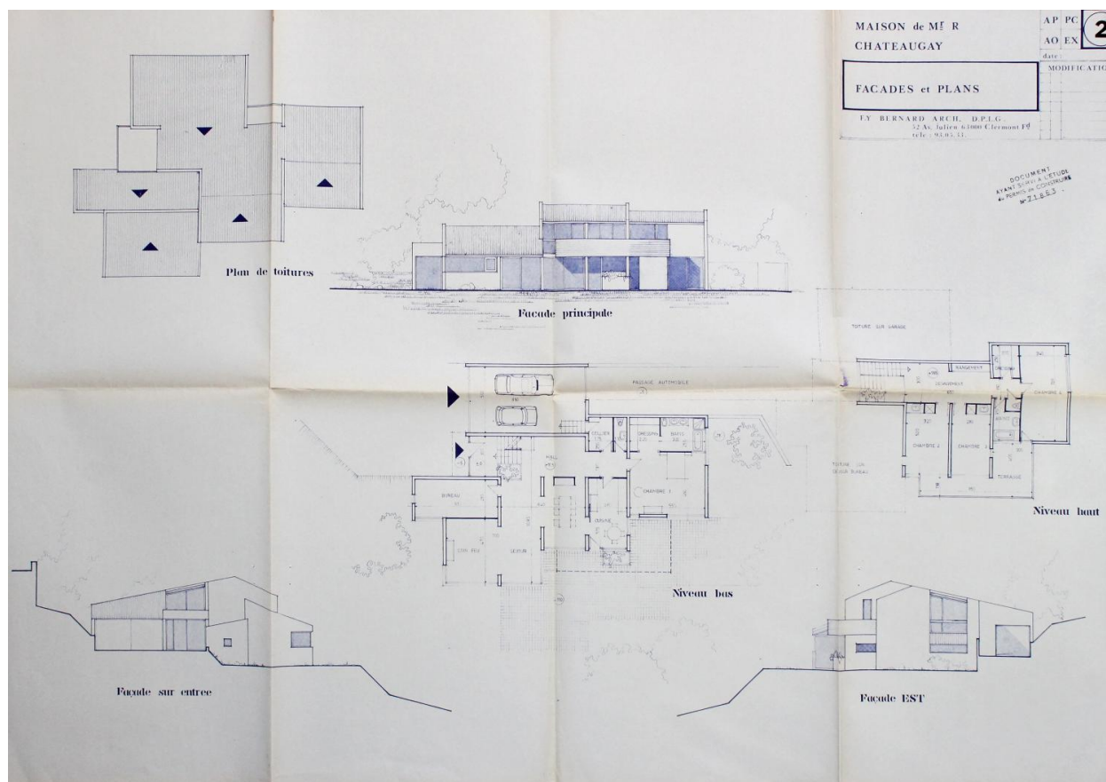
Châteaugay, la Maison R., plans des niveaux bas et haut, façades sud, est et ouest, François-Yves BERNARD architecte, 1975 (Archives municipales de Châteaugay).
