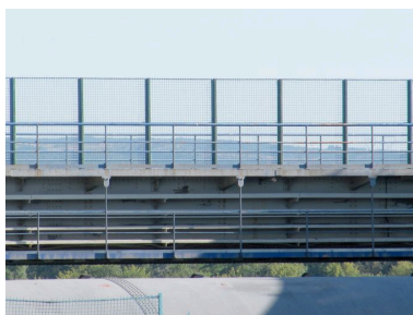
Parapet et tablier du pont, vue partielle (depuis la rive droite) Phot. I. Havard IVR82_20102600093NUCA
