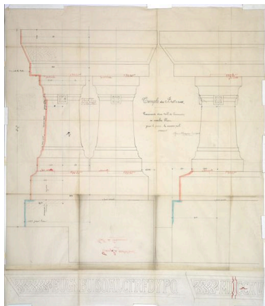
Dessin d'exécution pour la table Repro. Didier Gourbin, Autr. Gaspard André IVR82_20106906101NUCA
