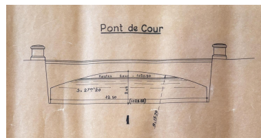
Plan de profils en travers du pont de Cour. 1943 (AD Haute-Savoie : 2478 W 172) Autr. Samir Mahfoudi IVR84_20257401338NUCA
