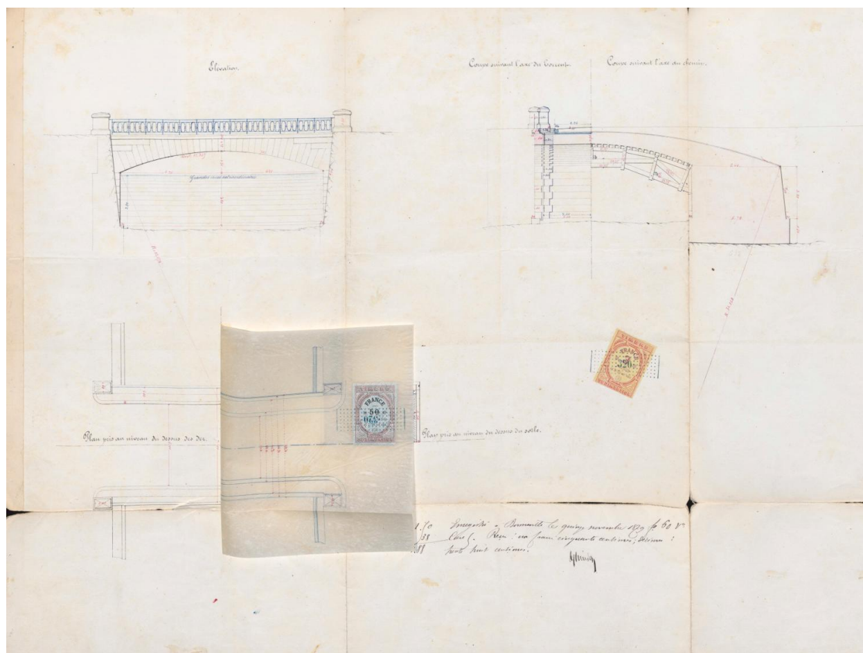
Construction d'un pont sur l'Arve, épure. 1870 (AD Haute-Savoie : 3 O 2511)
