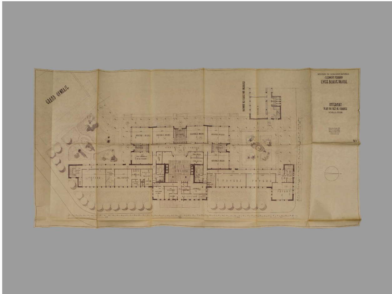
Internat, plan du rez-de-chaussée, 10/2/1953. (Plan tramé à 1, 75 m en application de la circulaire du 1/9/1952). (AC Clermont-Ferrand. 477 W 2.)
