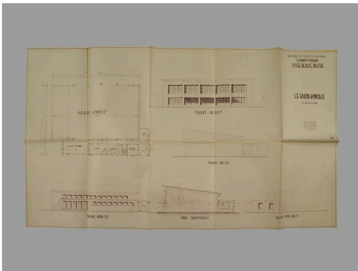
Grand gymnase, plan, coupe et 4 façades, 10/2/1953. (AC Clermont-Ferrand : 477 W 2.)
