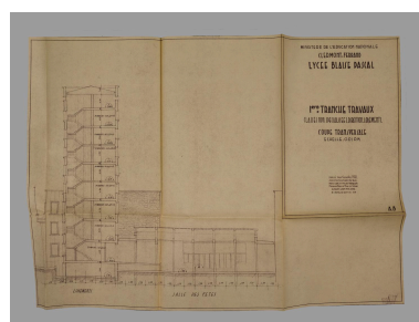
Première tranche des travaux. Coupe transversale, 25/11/1952. (AC Clermont-Ferrand : 477 W 2.) Repro. Christian Parisey, Autr. Georges Marie Noël IVR84_20206300560NUC4A
