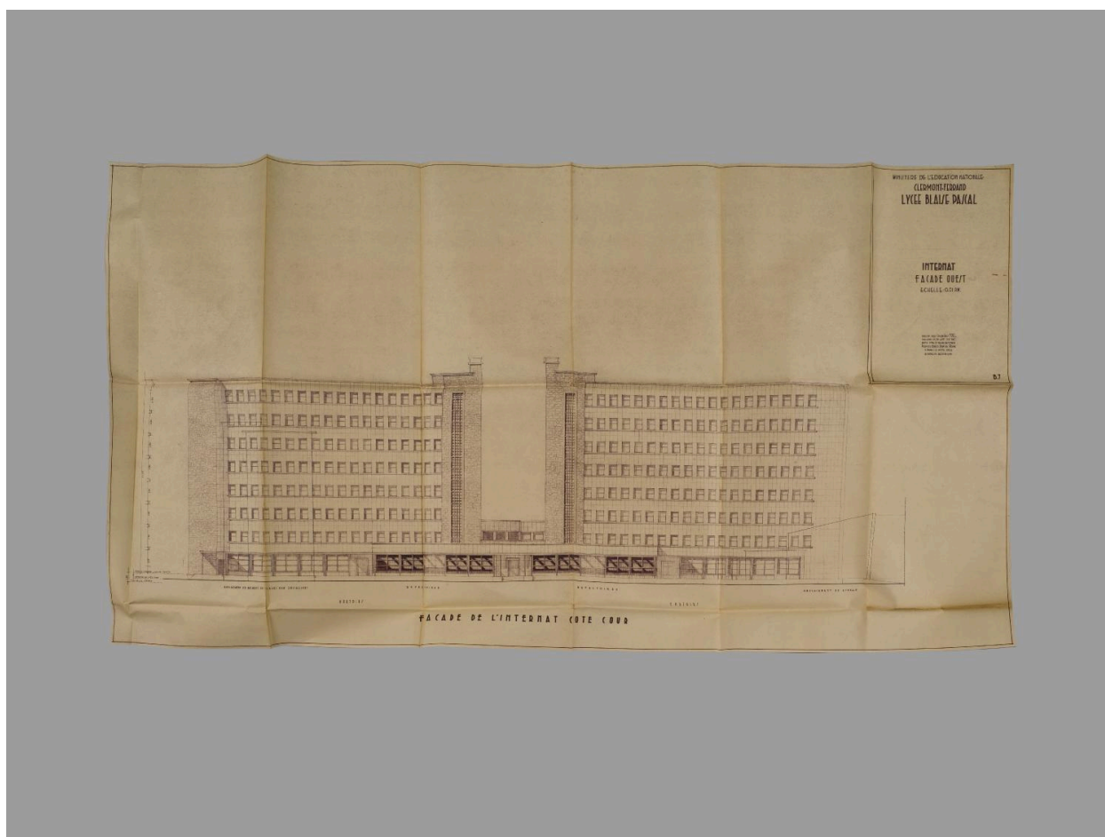
Internat, façade ouest, 10/2/1953. (AC Clermont-Ferrand : 477 W 2.)
