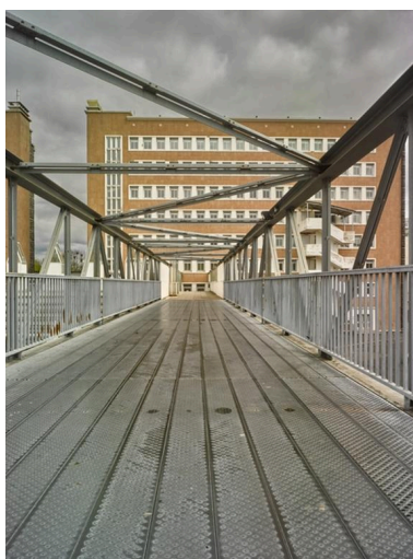
Depuis la passerelle vers l'est : façade du bâtiment d'internat sud. Phot. Christian Parisey IVR84_20196300061NUC4A
