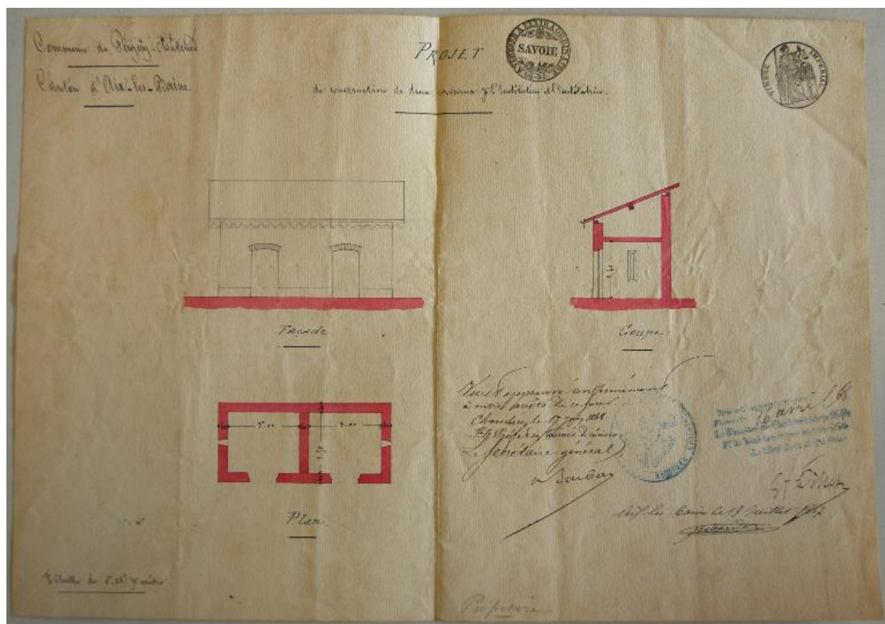
AD 72. Projet de construction de deux caveaux pour les instituteurs, 1867
