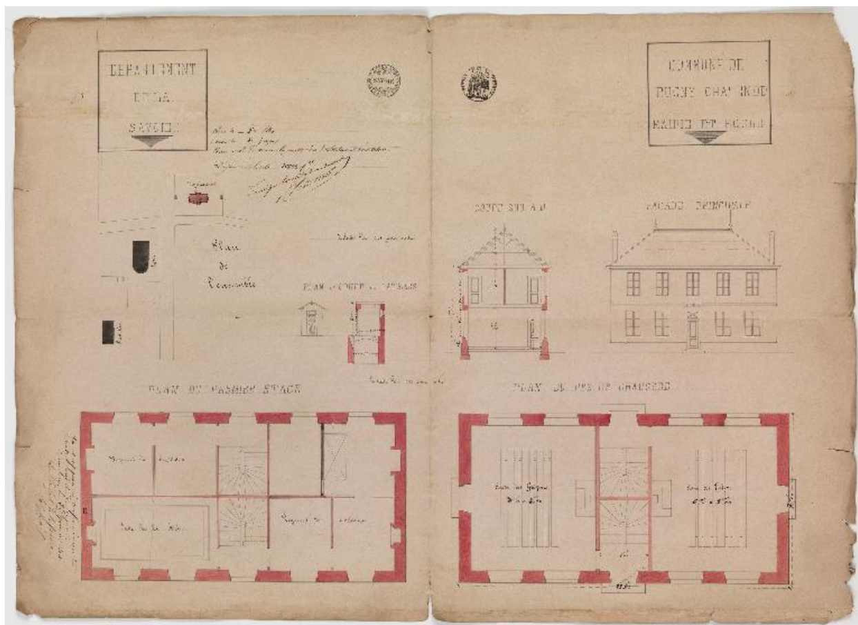
AD 73. Plans, coupes, élévation école-mairie. 1864
