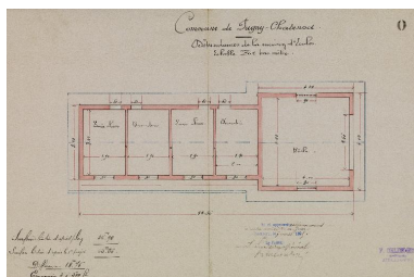
AD 72. Maison d'écoles. Dépendance : plan du rez-de-chaussée. 1895. Phot. Thierry Leroy IVR84_20177301732NUCA
