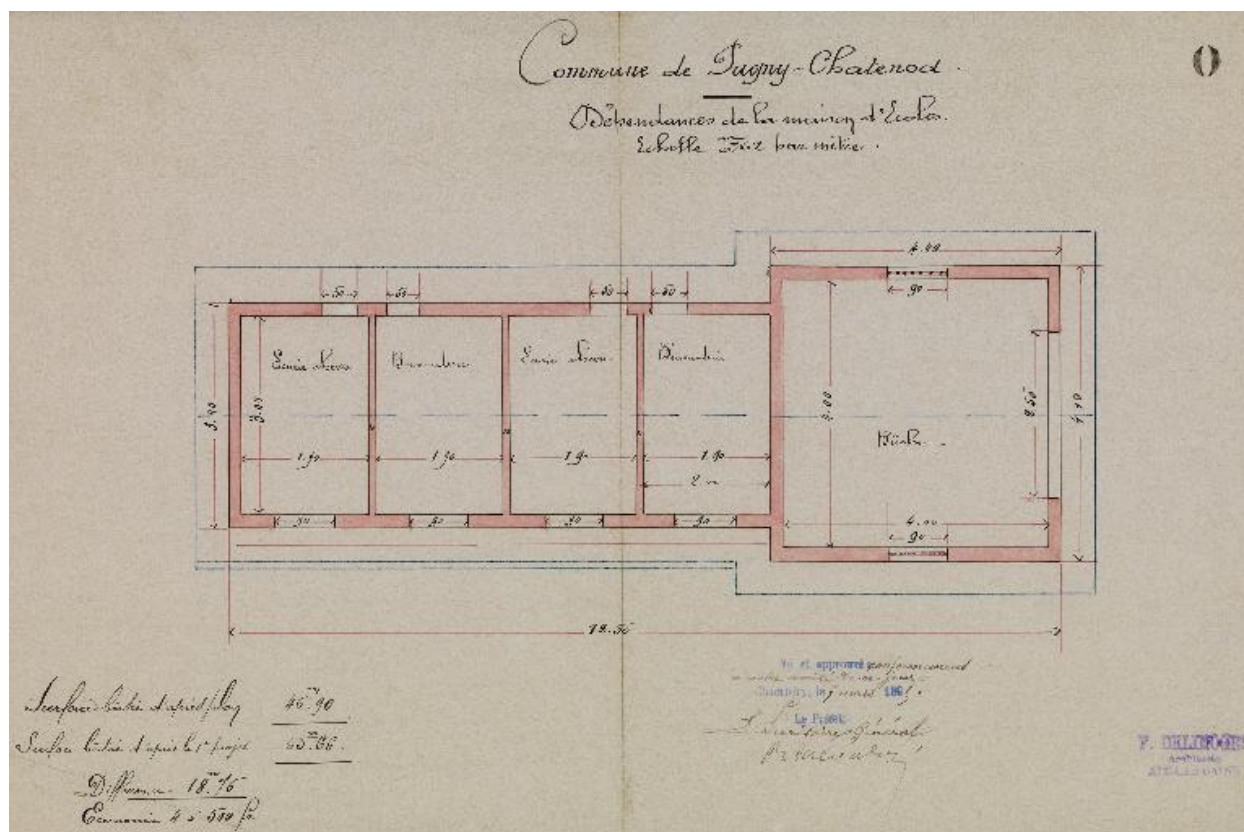
AD 72. Maison d'écoles. Dépendance : plan du rez-de-chaussée. 1895.
