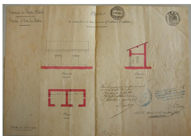
AD 72. Projet de construction de deux caveaux pour les instituteurs, 1867 Phot. Thierry Monnet IVR84_20177300794NUCA
