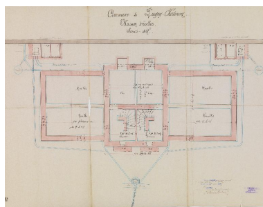
AD 72. Maison d'écoles, plan du sous-sol. 1895 Phot. Thierry Leroy IVR84_20177301724NUCA
