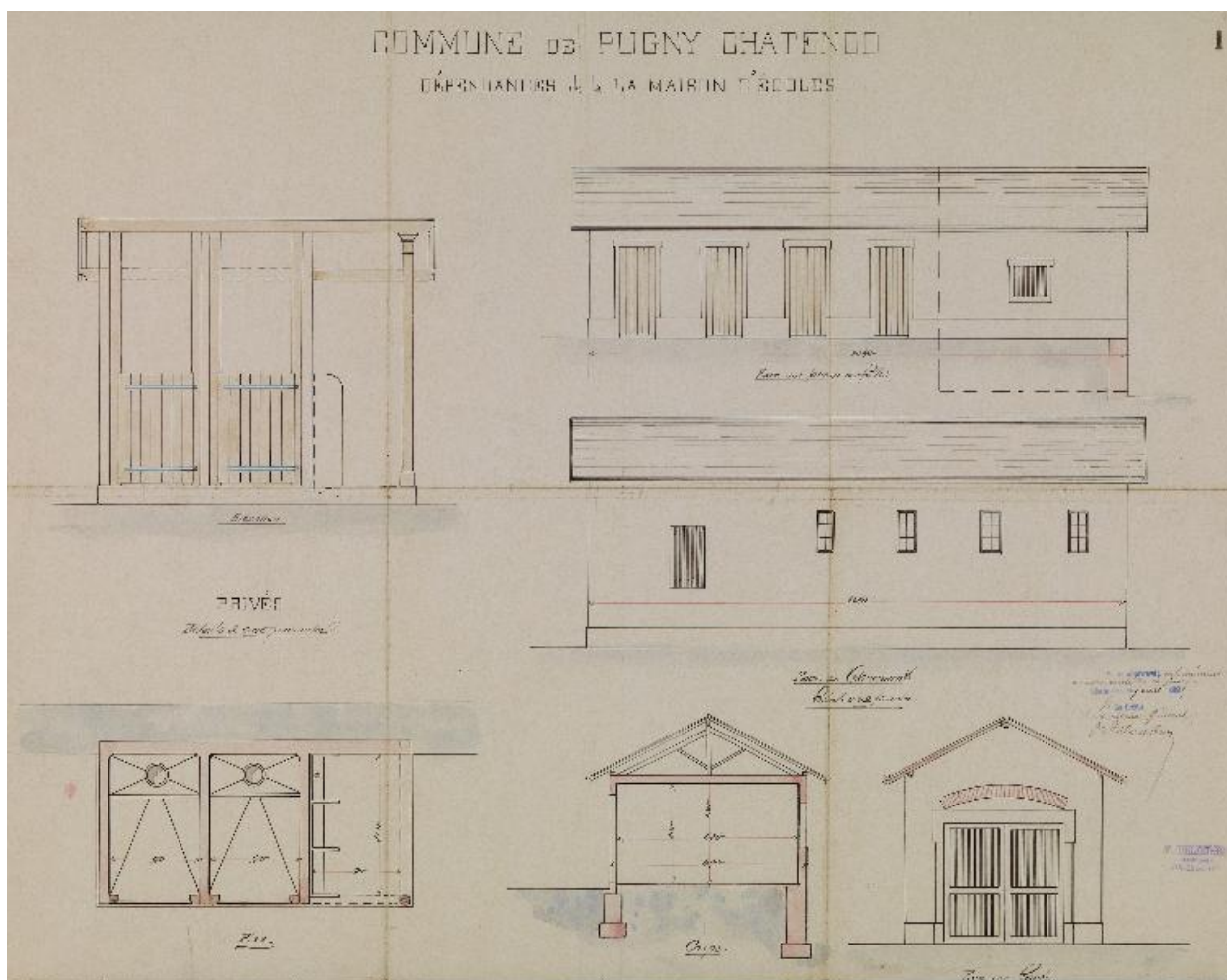
AD 73. Maison d'écoles. Dépendances : plans, élévations, coupes. 1895.
