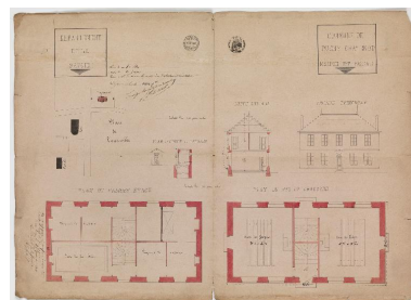
AD 73. Plans, coupes, élévation école-mairie. 1864 Phot. Thierry Leroy IVR84_20177301718NUCA
