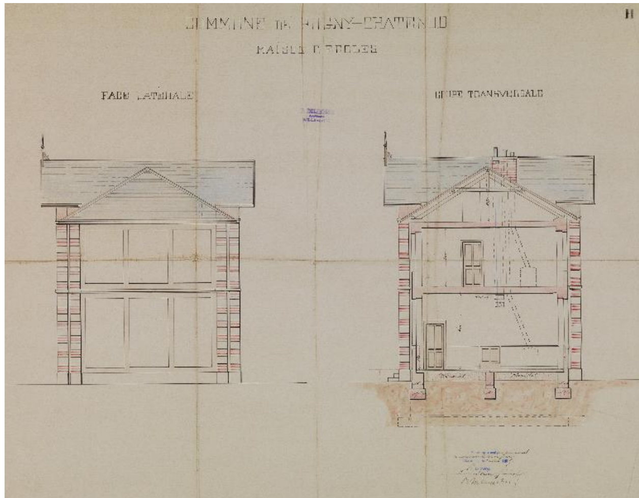
AD 73. Maison d'écoles, coupes sur la face latérale et transversale. 1895.
