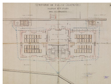
AD 73. Maison d'écoles, plan du rez-de-chaussée. 1895 Phot. Thierry Leroy IVR84_20177301725NUCA
