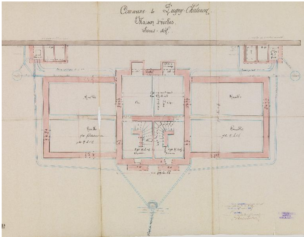
AD 72. Maison d'écoles, plan du sous-sol. 1895
