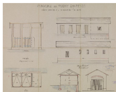
AD 73. Maison d'écoles. Dépendances : plans, élévations, coupes. 1895. Phot. Thierry Leroy IVR84_20177301731NUCA
