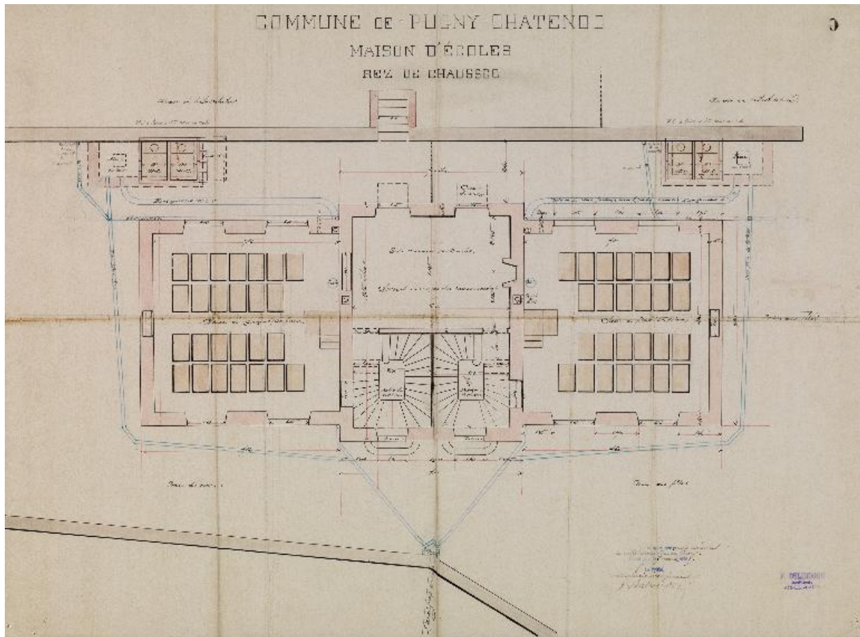
AD 73. Maison d'écoles, plan du rez-de-chaussée. 1895
