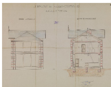
AD 73. Maison d'écoles, coupes sur la face latérale et transversale. 1895. Phot. Thierry Leroy IVR84_20177301730NUCA
