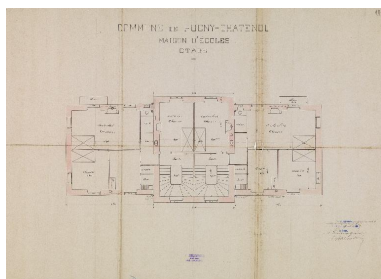
Ad 73. Maison d'écoles, plan de l'étage. 1895 Phot. Thierry Leroy IVR84_20177301726NUCA
