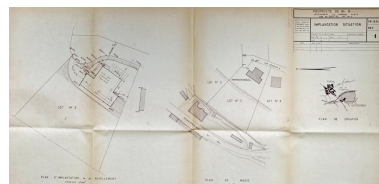
Durtol, la maison Br.*, plan de situation et de masse, 1967, Julien Arnaud et Robert Bournadet architectes (archives municipales de Durtol). Repro. Christophe Laurent, Autr. Julien Arnaud, Autr. R. Bournadet IVR84_20246301949NUCA
