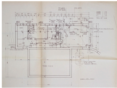
Durtol, la maison Br.*, plan du sous-sol, 1967, Julien Arnaud et Robert Bournadet architectes (archives municipales de Durtol). Repro. Christophe Laurent, Autr. Julien Arnaud, Autr. R. Bournadet IVR84_20246301950NUCA
