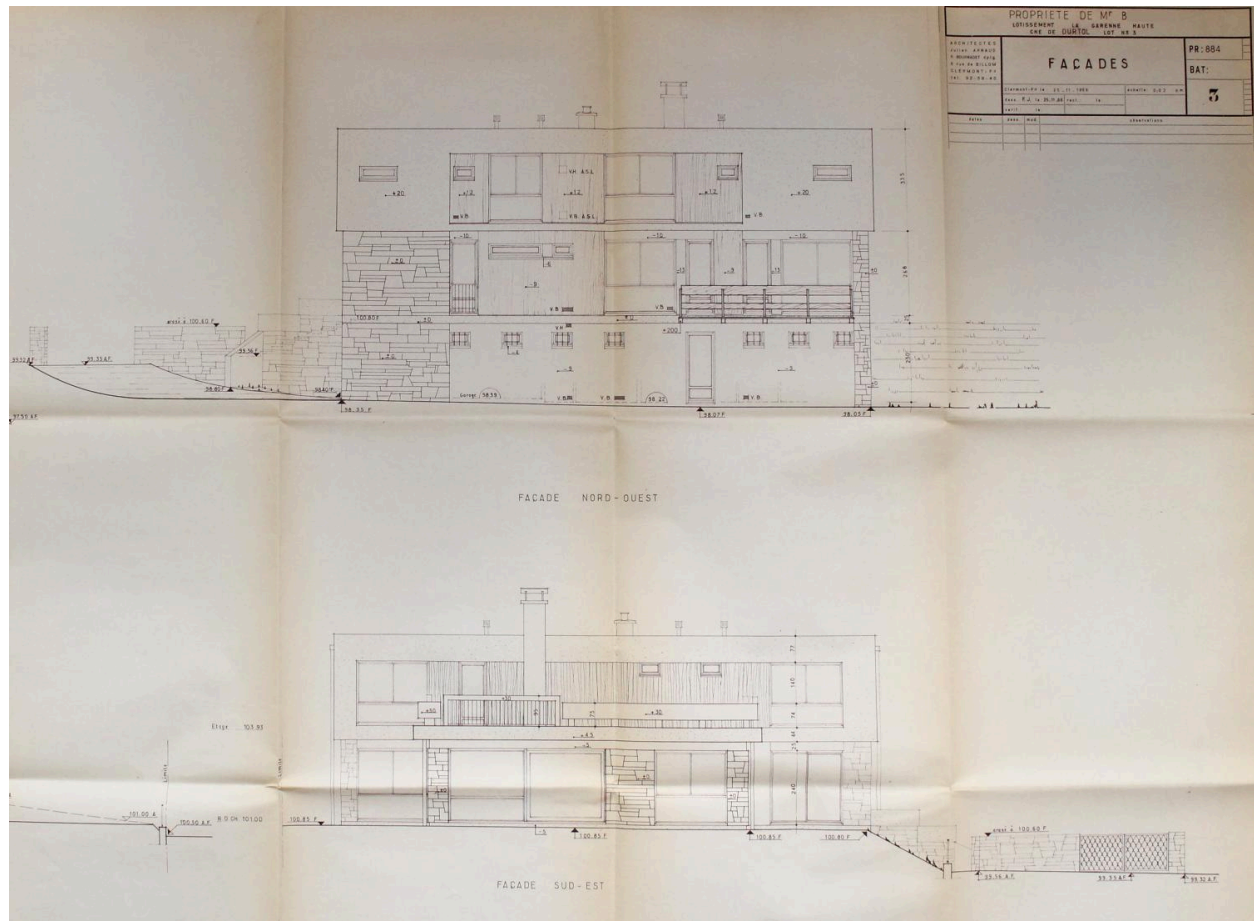
Durtol, la maison Br.*, façade principale et façade postérieure, 1967, Julien Arnaud et Robert Bournadet architectes (archives municipales de Durtol).
