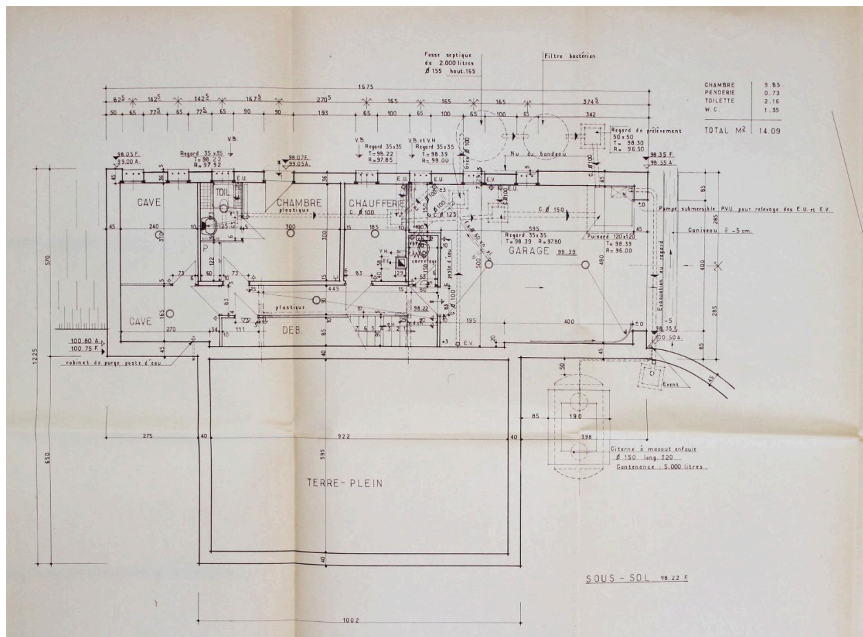
Durtol, la maison Br.*, plan du sous-sol, 1967, Julien Arnaud et Robert Bournadet architectes (archives municipales de Durtol).
