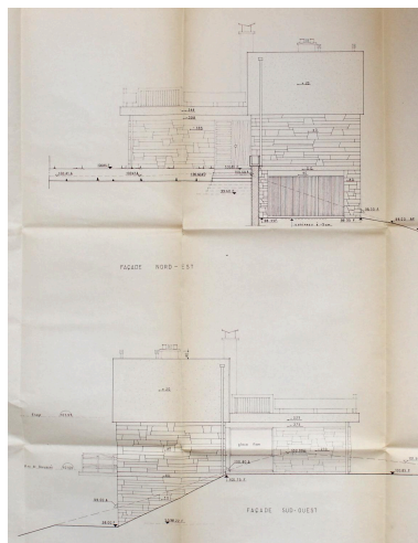
Durtol, la maison Br.*, façades latérales, 1967, Julien Arnaud et Robert Bournadet architectes (archives municipales de Durtol). Repro. Christophe Laurent, Autr. Julien Arnaud, Autr. R. Bournadet IVR84_20246301954NUCA
