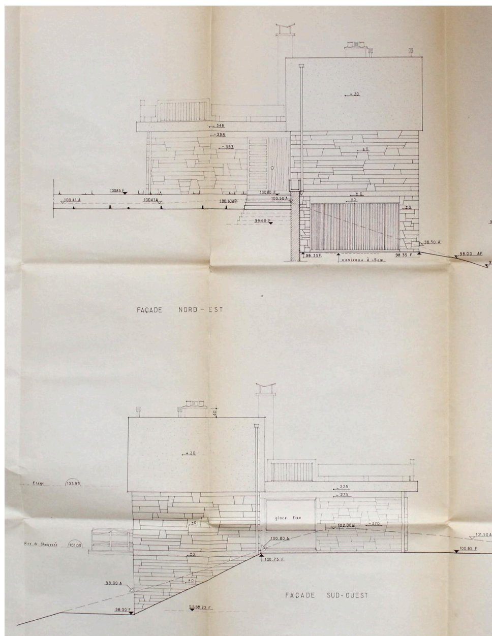
Durtol, la maison Br.*, façades latérales, 1967, Julien Arnaud et Robert Bournadet architectes (archives municipales de Durtol).
