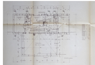
Durtol, la maison Br.*, plan de l'étage, 1967, Julien Arnaud et Robert Bournadet architectes (archives municipales de Durtol). Repro. Christophe Laurent, Autr. Julien Arnaud, Autr. R. Bournadet IVR84_20246301952NUCA
