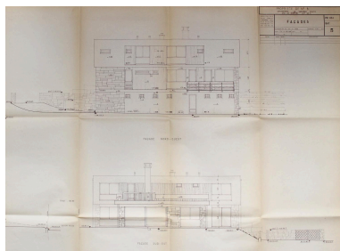
Durtol, la maison Br.*, façade principale et façade postérieure, 1967, Julien Arnaud et Robert Bournadet architectes (archives municipales de Durtol). Repro. Christophe Laurent, Autr. Julien Arnaud, Autr. R. Bournadet IVR84_20246301953NUCA
