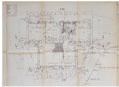
Durtol, la maison Br.*, plan du rez-de-chaussée, 1967, Julien Arnaud et Robert Bournadet architectes (archives municipales de Durtol). Repro. Christophe Laurent, Autr. Julien Arnaud, Autr. R. Bournadet IVR84_20246301951NUCA
