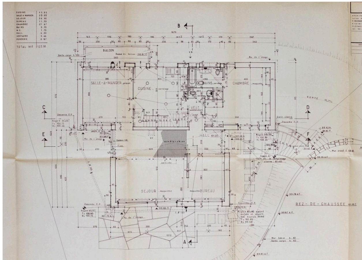
Durtol, la maison Br.*, plan du rez-de-chaussée, 1967, Julien Arnaud et Robert Bournadet architectes (archives municipales de Durtol).
