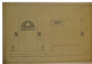
Elévations du tombeau de la famille Petit prévu pour le cimetière de Miribel, calque [1934 ?] : le modèle est très proche du monument élevé pour la famille Boretti Phot. Véronique (reproduction) Belle IVR84_20196900293NUCA
