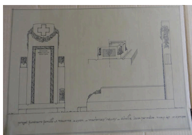
Elévations du tombeau de la famille J. Trotte, Tony Vialy dessinateur, calque, 1935 Phot. Véronique (reproduction) Belle IVR84_20196900294NUCA
