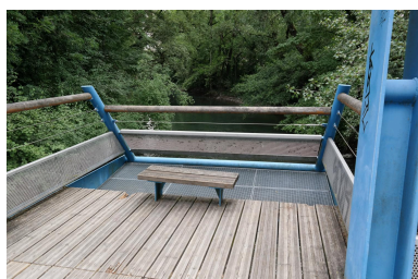
Passerelle piétonne sur le Thiou, détail d'un bélevédère en porte-à-faux Phot. Pascale Renard IVR84_20207403845NUCA
