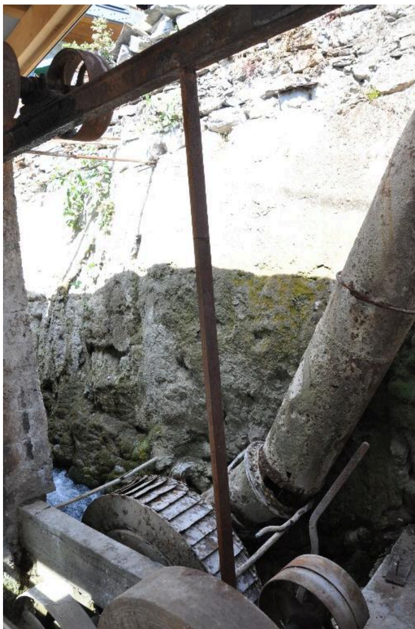
Vue de la petite roue hydraulique et d'un tronçon de conduite, 2014.
