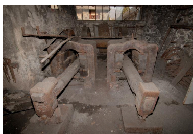
Vue des martinets, 2011. Phot. Jean-François Laurenceau IVR82_20157301639NUCA
