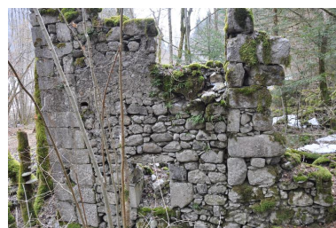
Elevation du mur nord-ouest du moulin. Phot. Clara Bérelle IVR82_20137301615NUCA
