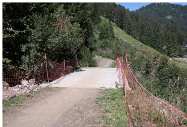
Passerelle VTT de Plaine Dranse, vue du tablier Phot. Pascale Renard IVR84_20207401421NUCA
