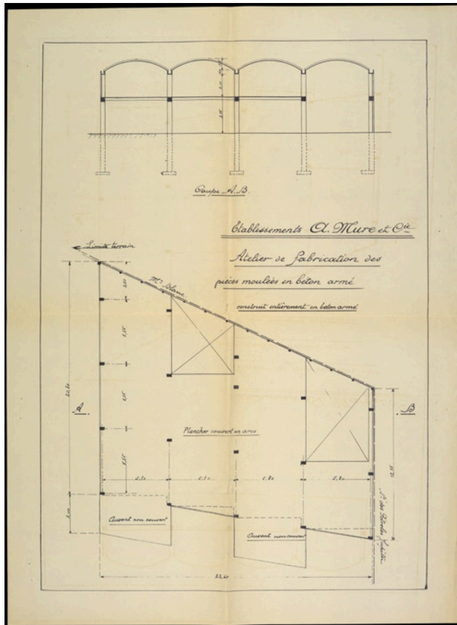
Coupe AB atelier de fabrication des Ets Mûre
