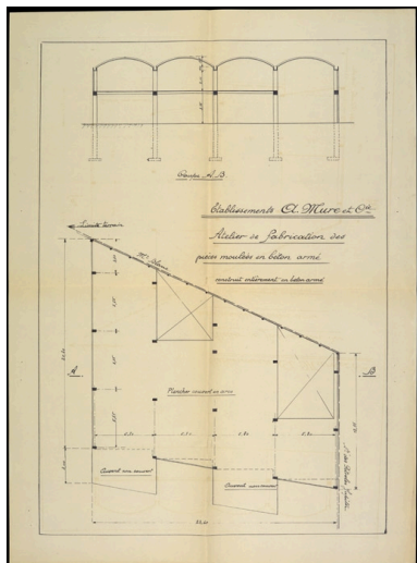
Coupe AB atelier de fabrication des Ets Mûre Repro. Gilles Bernasconi IVR82_20086901863NUCB
